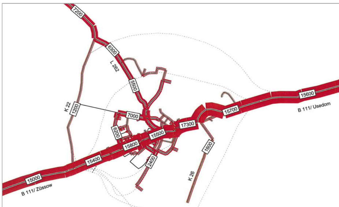
Abbildung 1: Prognoseverkehrsmengen DTV 2020 – Prognose-Nullfall (Ohne-Fall)
