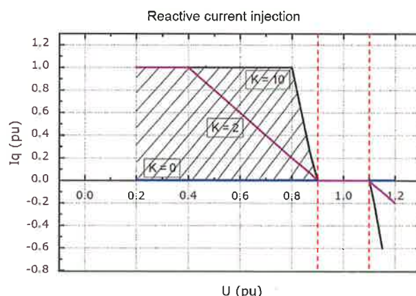
Abbildung 10-6: Blindstromeinspeisung
