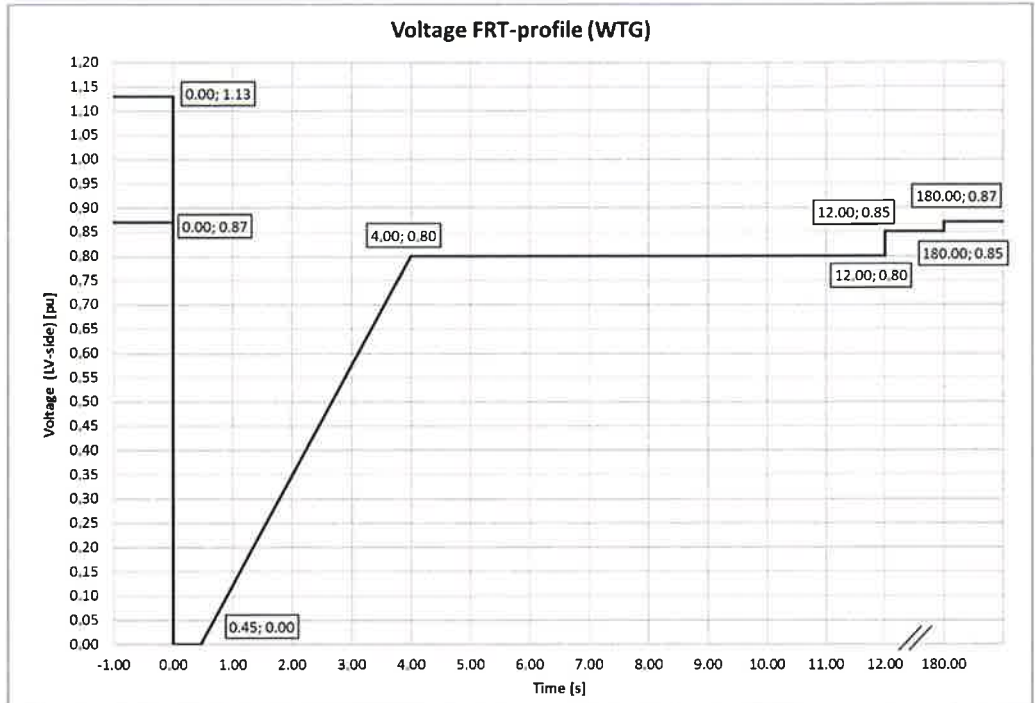
Abbildung 10-5: Niedrige Spannungstoleranzkurve für symmetrische und asymmetrische Störungen, wobei U die gemessene Spannung im Stromnetz darstellt.
