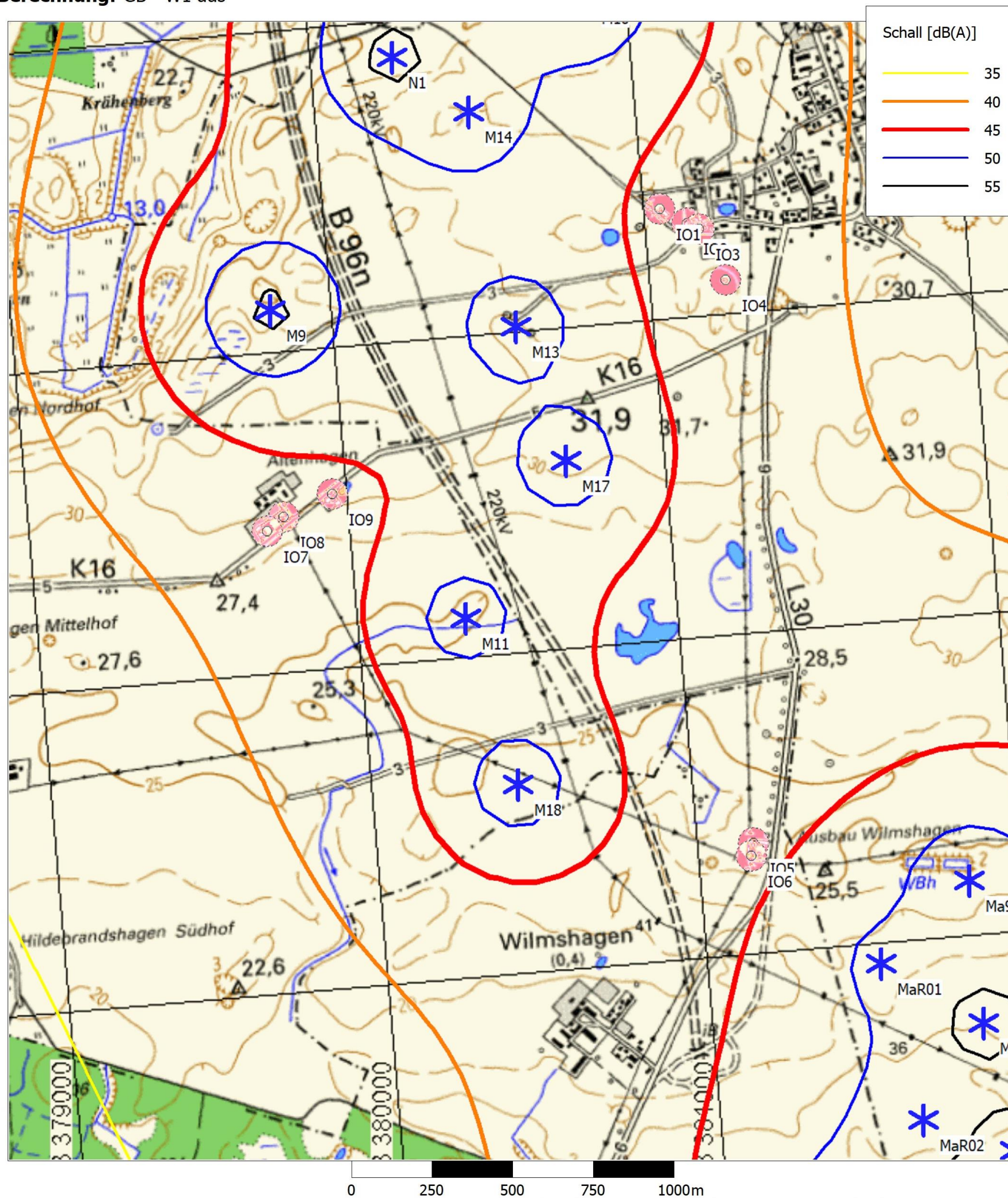
Karte: Miltzow MM, Maßstab 1:17,500, Mitte: Germany UTM ETRS89 Zone: 33 Ost: 3,380,639 Nord: 6,005,327 * Existierende WEA ■ Schall-Immissionsort Schallberechnungs-Modell: ISO 9613-2 Deutschland (Interimsverfahren). Windgeschwindigkeit: Lautester Wert bis 95% Nennleistung Höhe über Meeresspiegel von aktivem Höhenlinien-Objekt
