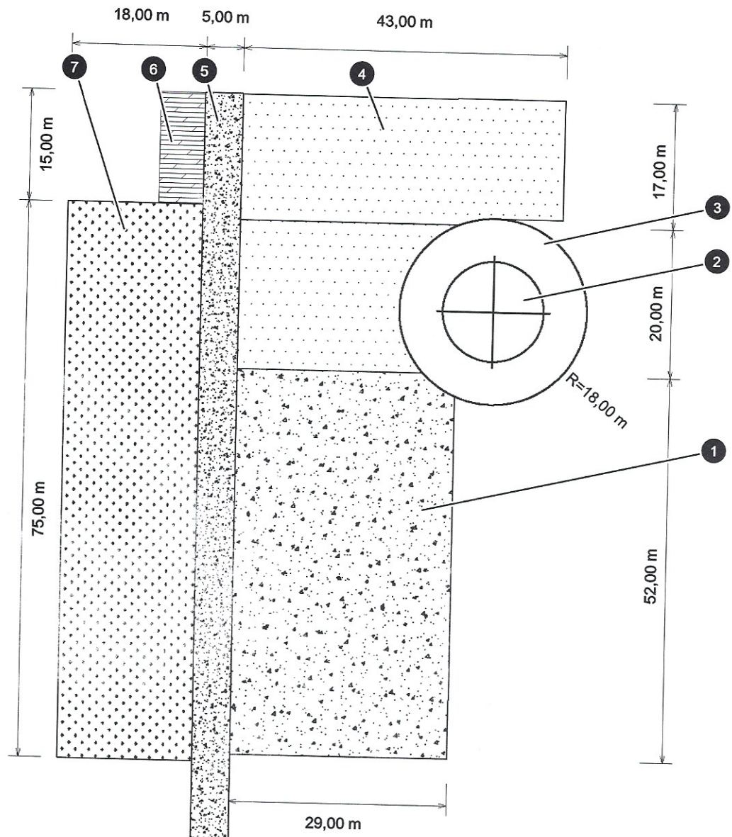
Abb. 8: Baustellenfläche Baumaße
