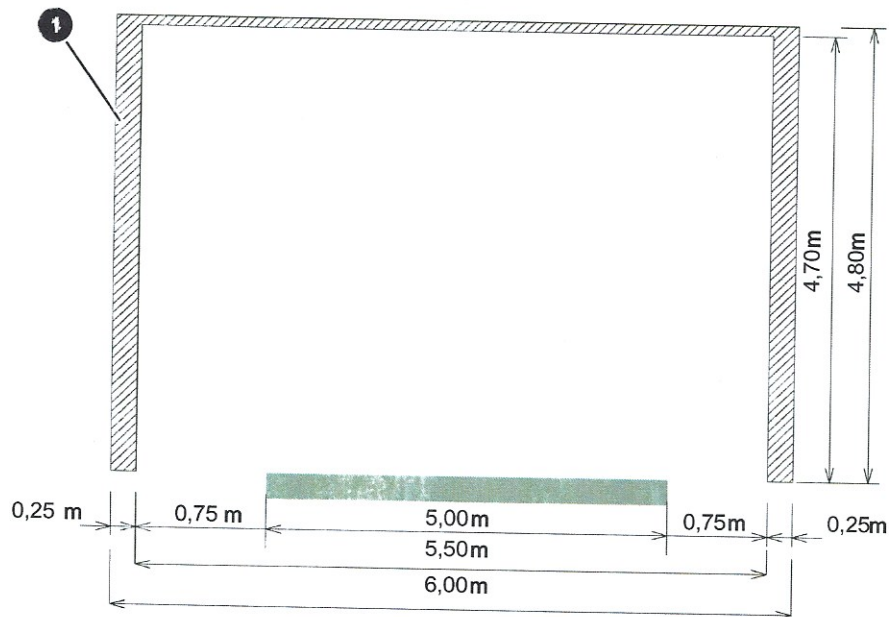
Abb. 5: Lichtraumprofil
