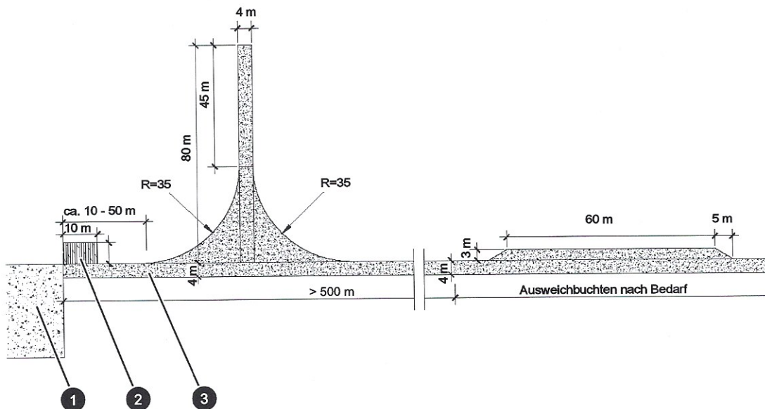
Abb. 1: Trassierungselemente
