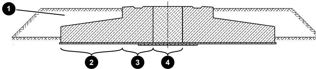
Abb. 1: Fundamentschnitt mit Aufsüttung
