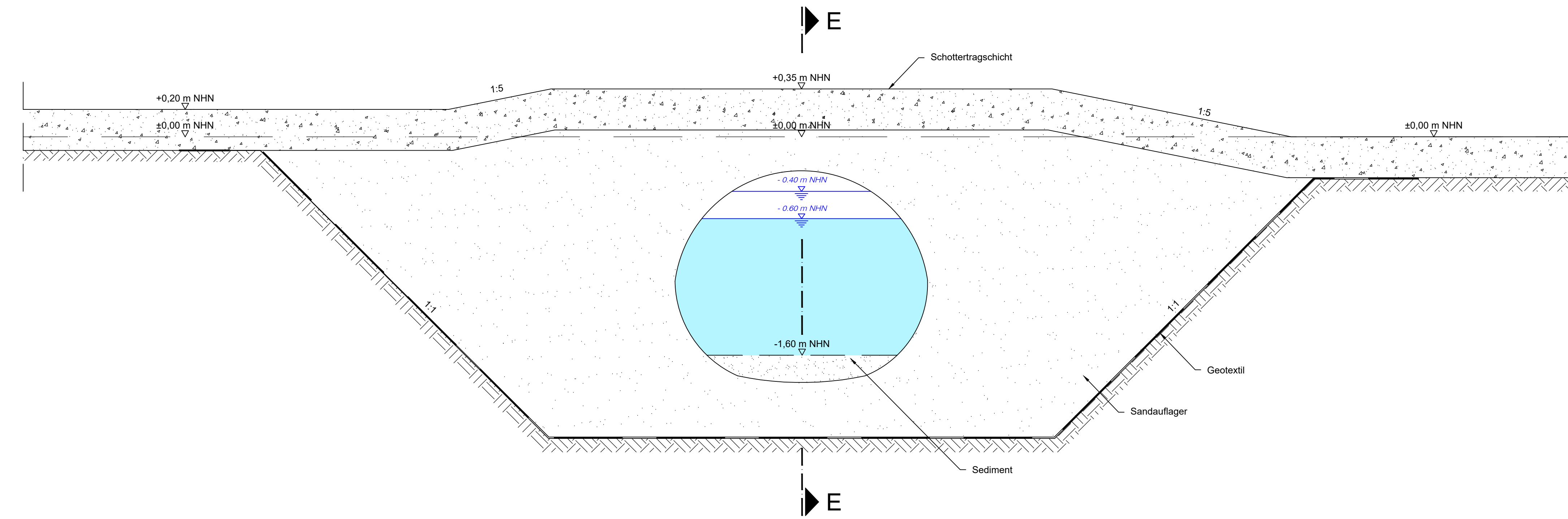
Schnitt E-E (VS_DU_3)
