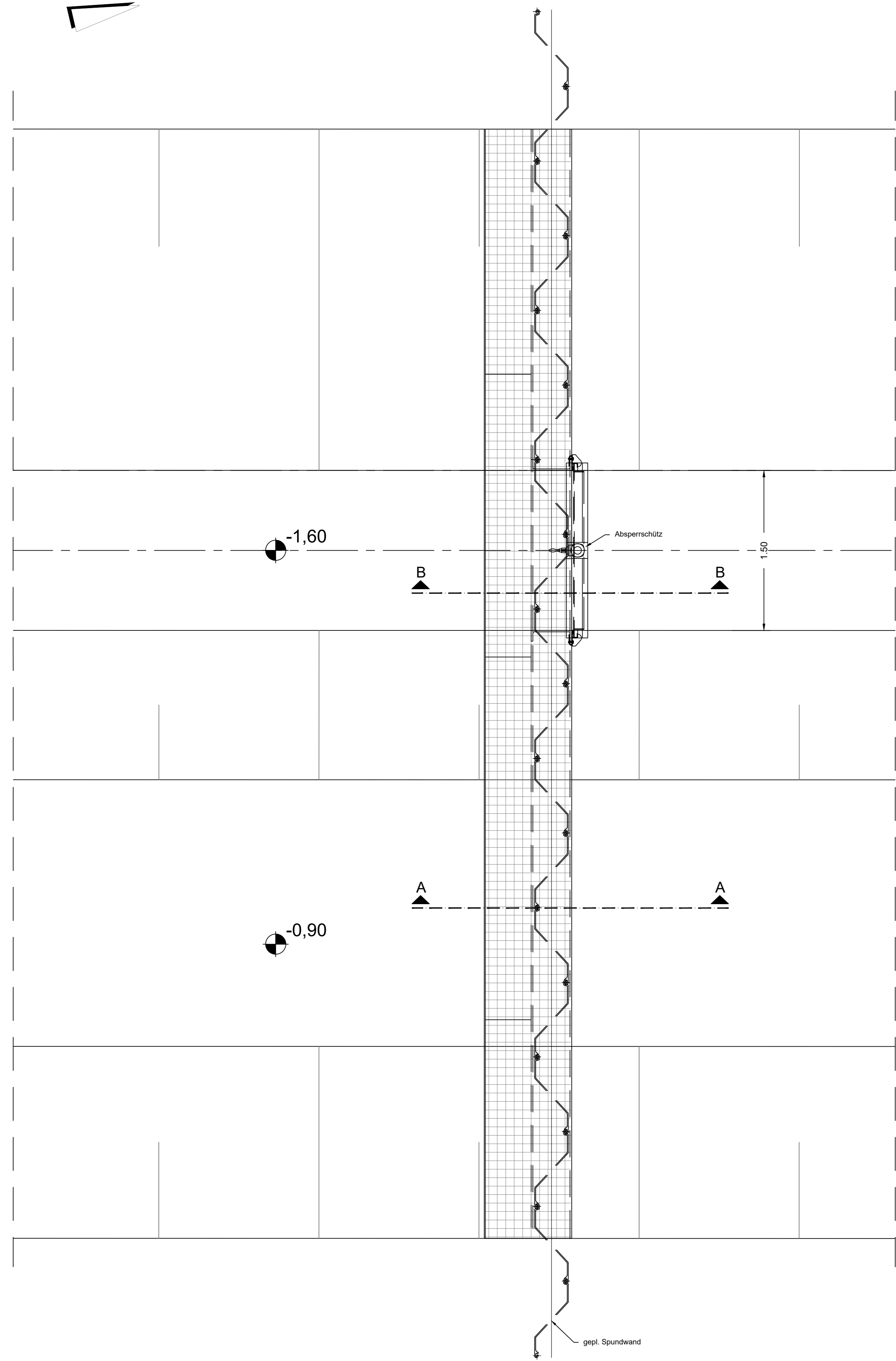
Draufsicht Spundwand 1+215 (NF_AS_1)
