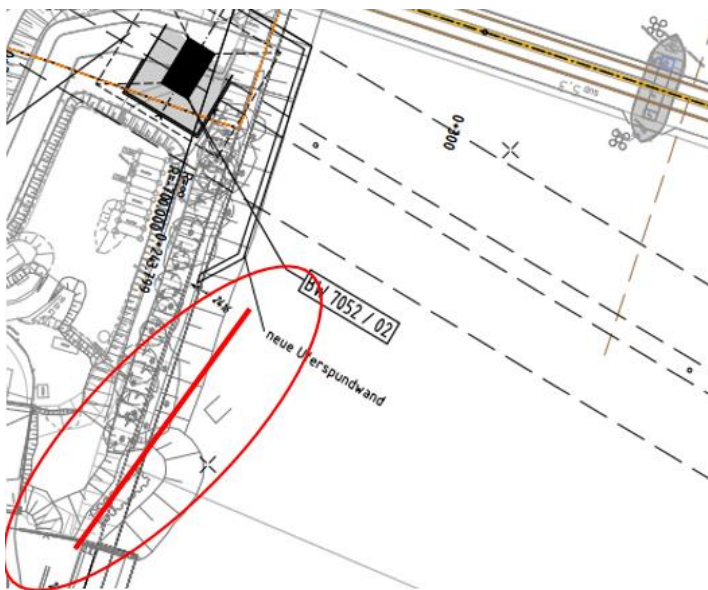
Abbildung 5: Lage des Auslassbauwerks für Fischrückführung
