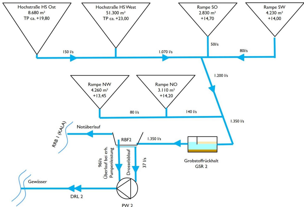
Abbildung 9: Fließschema im EA2 mit Abflüssen bei T = 5
