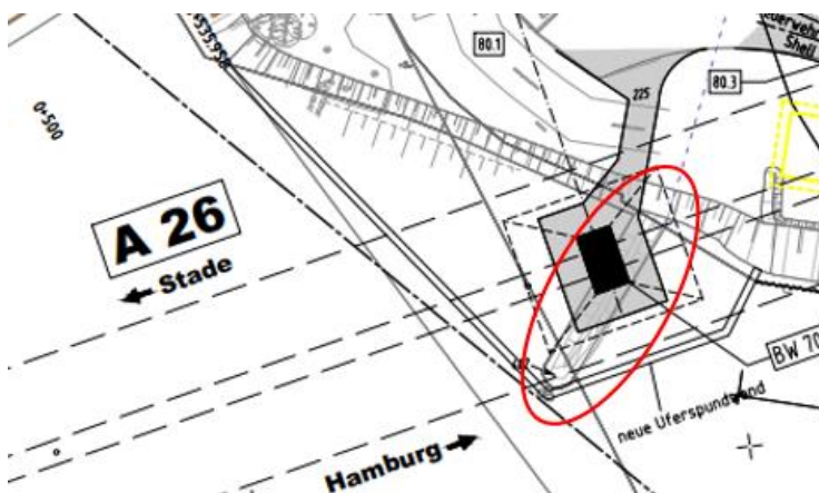
Abbildung 7: Lage der Anlagen im Bereich Hohe Schaar Hafen (Holzdalben, Fangedamm)
