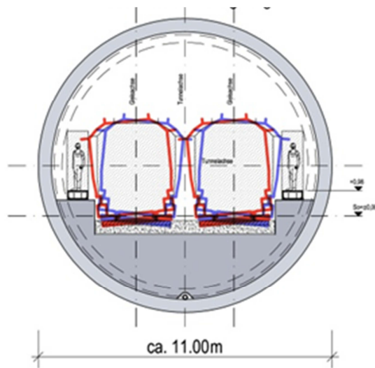
Abbildung 10: Systemquerschnitt Variante 1
