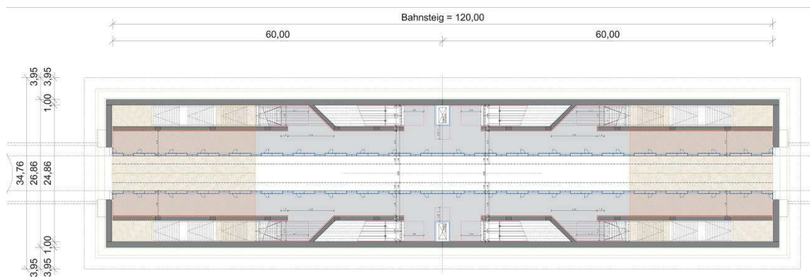
Abbildung 22: Haltestellentyp D
