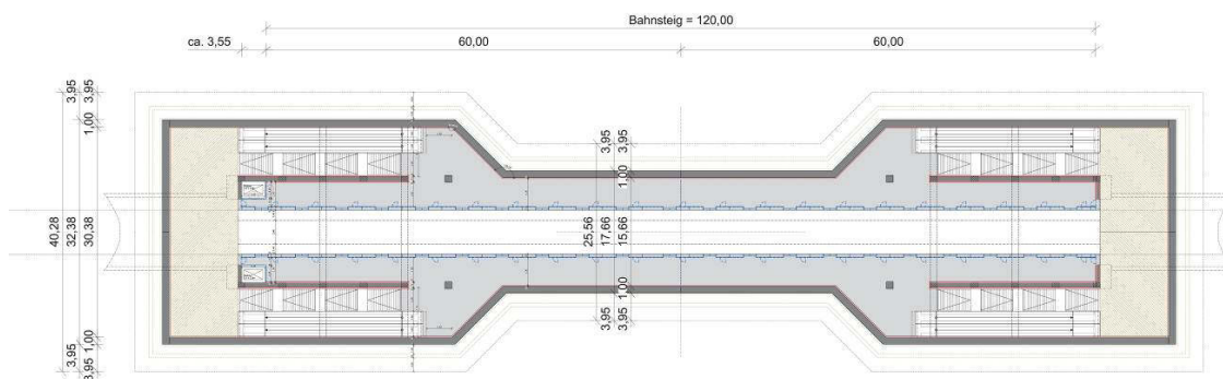
Abbildung 20: Haltestellentyp B
