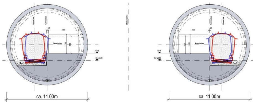
Abbildung 11: Systemquerschnitt Variante 2
