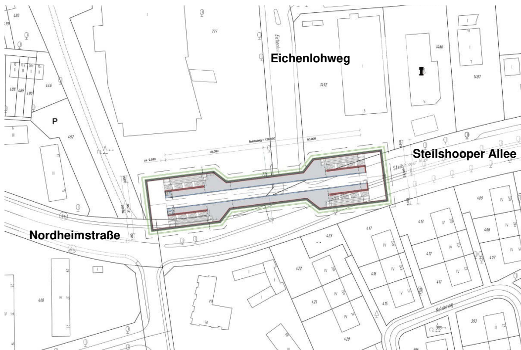
Abbildung 31: Lagevariante 2 "Eichenlohweg"
