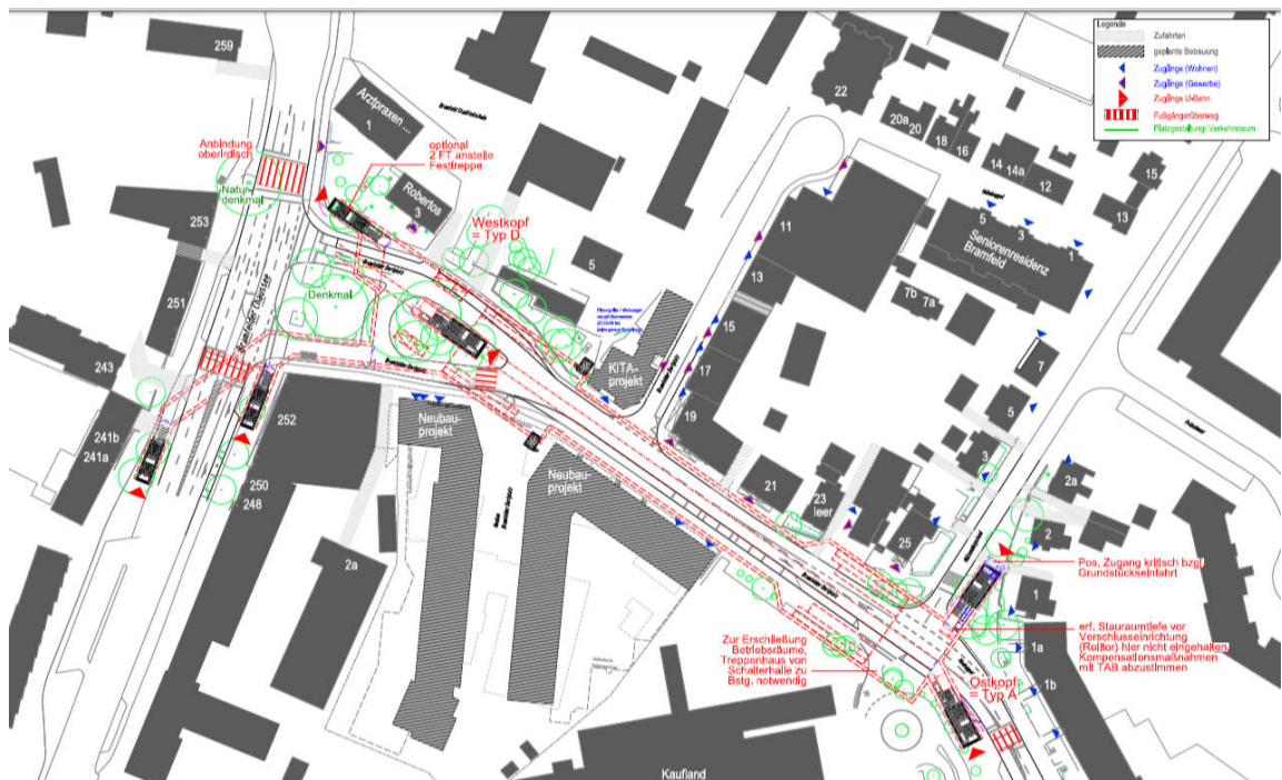
Abbildung 49: Darstellung Ausgänge Hst. BD – Variante mit Fußgängertunnel- Oberfläche
