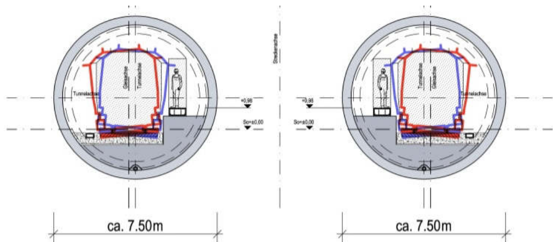
Abbildung 12: Systemquerschnitt Variante 3
