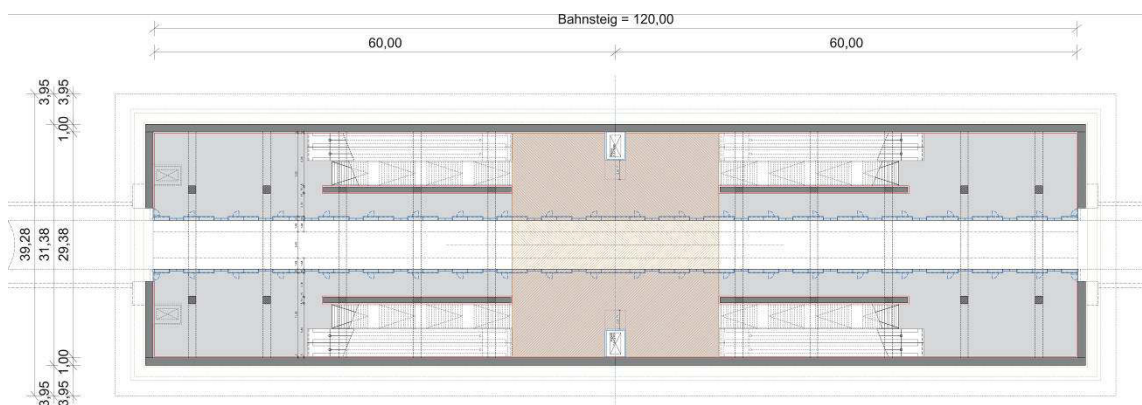
Abbildung 23: Haltestellentyp E
