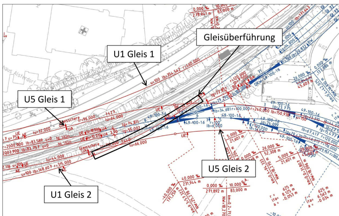
Abbildung 52: Gleisüberführung östlich Sengelmannstraße
