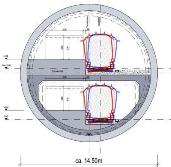
Abbildung 13: Systemquerschnitt Variante 4
