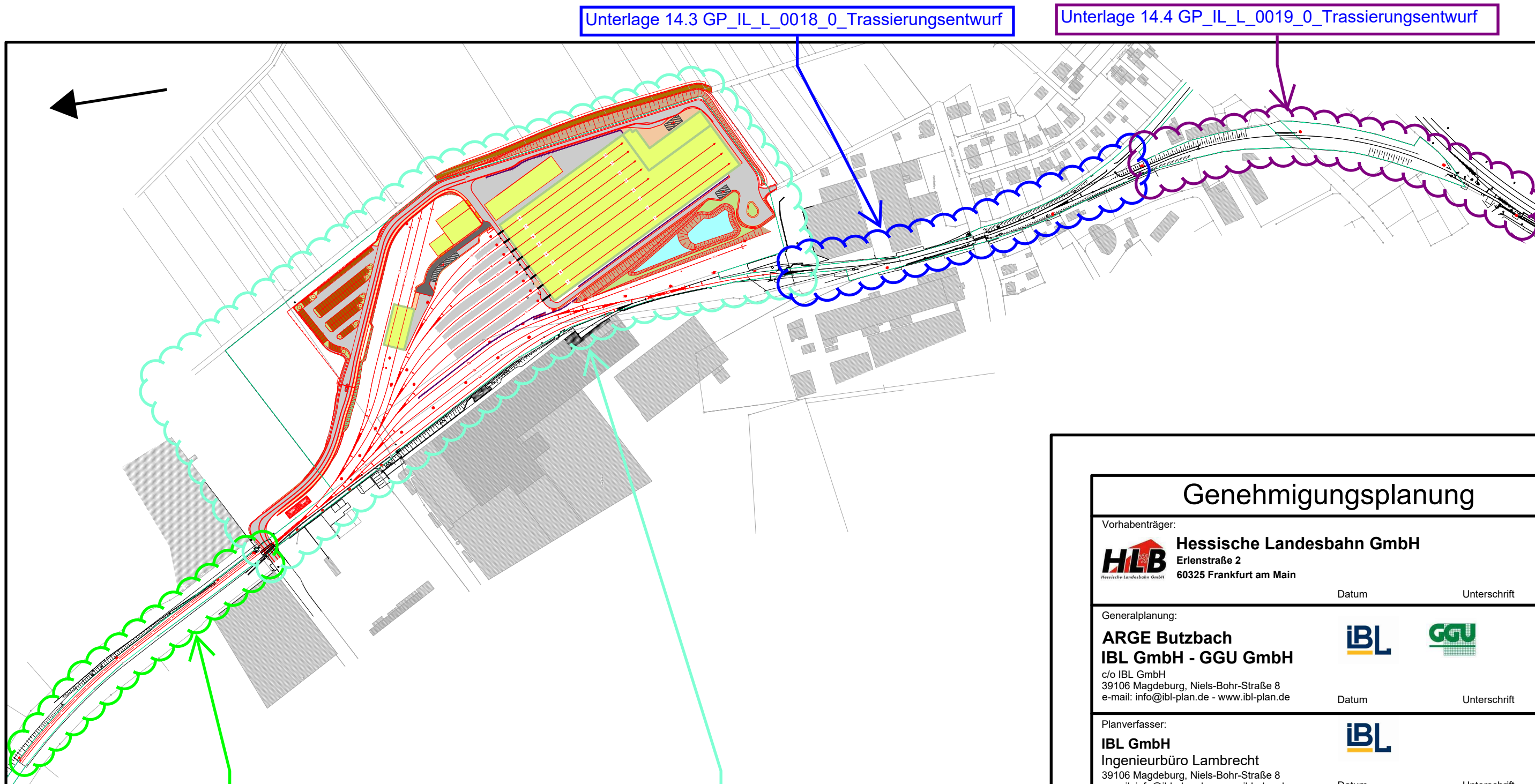
Unterlage 14.1 GP_IL_L_0016_0_Trassierungsentwurf
