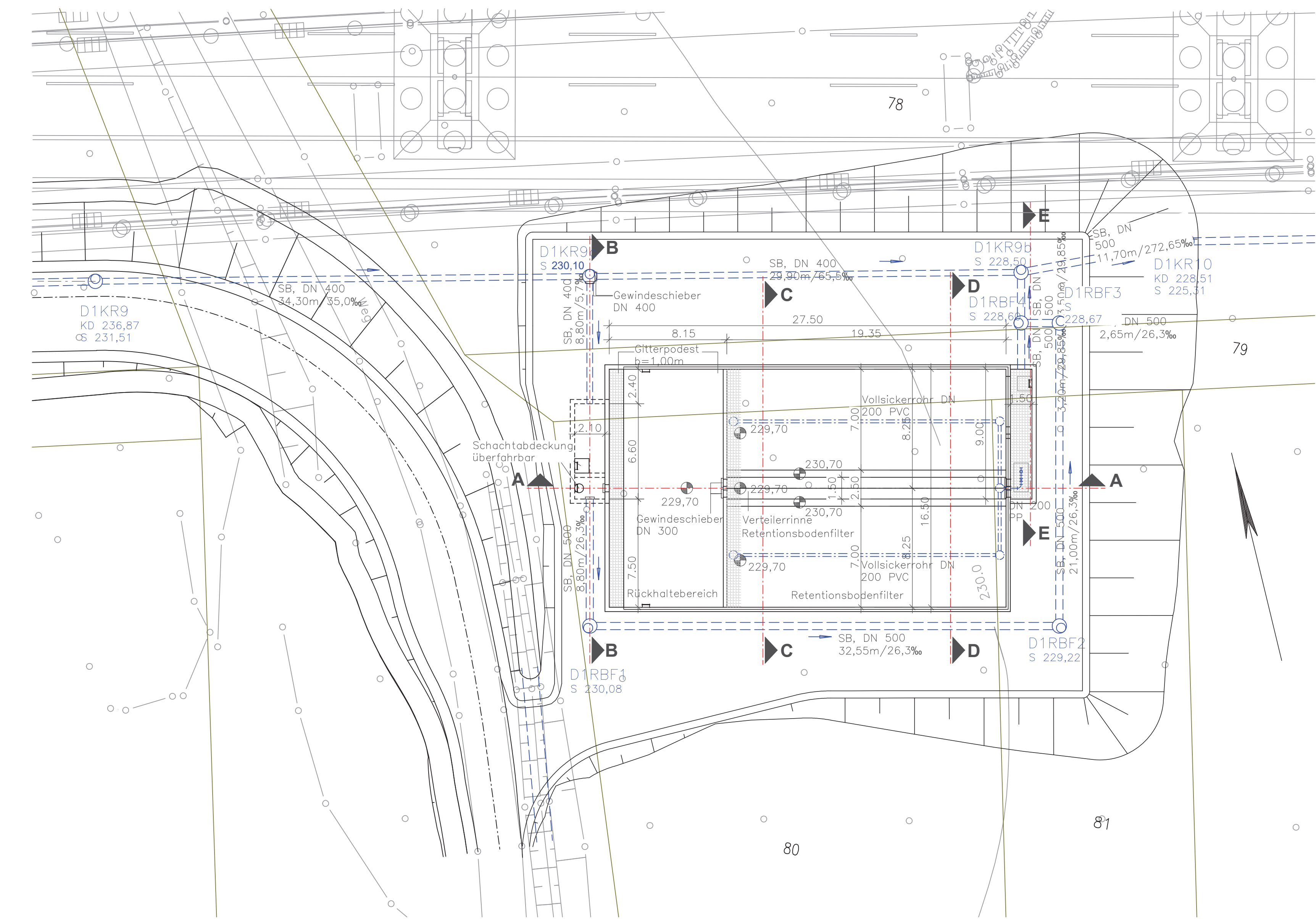
Draufsicht Retentionsfilterbecken 1 Maßstab 1:200
