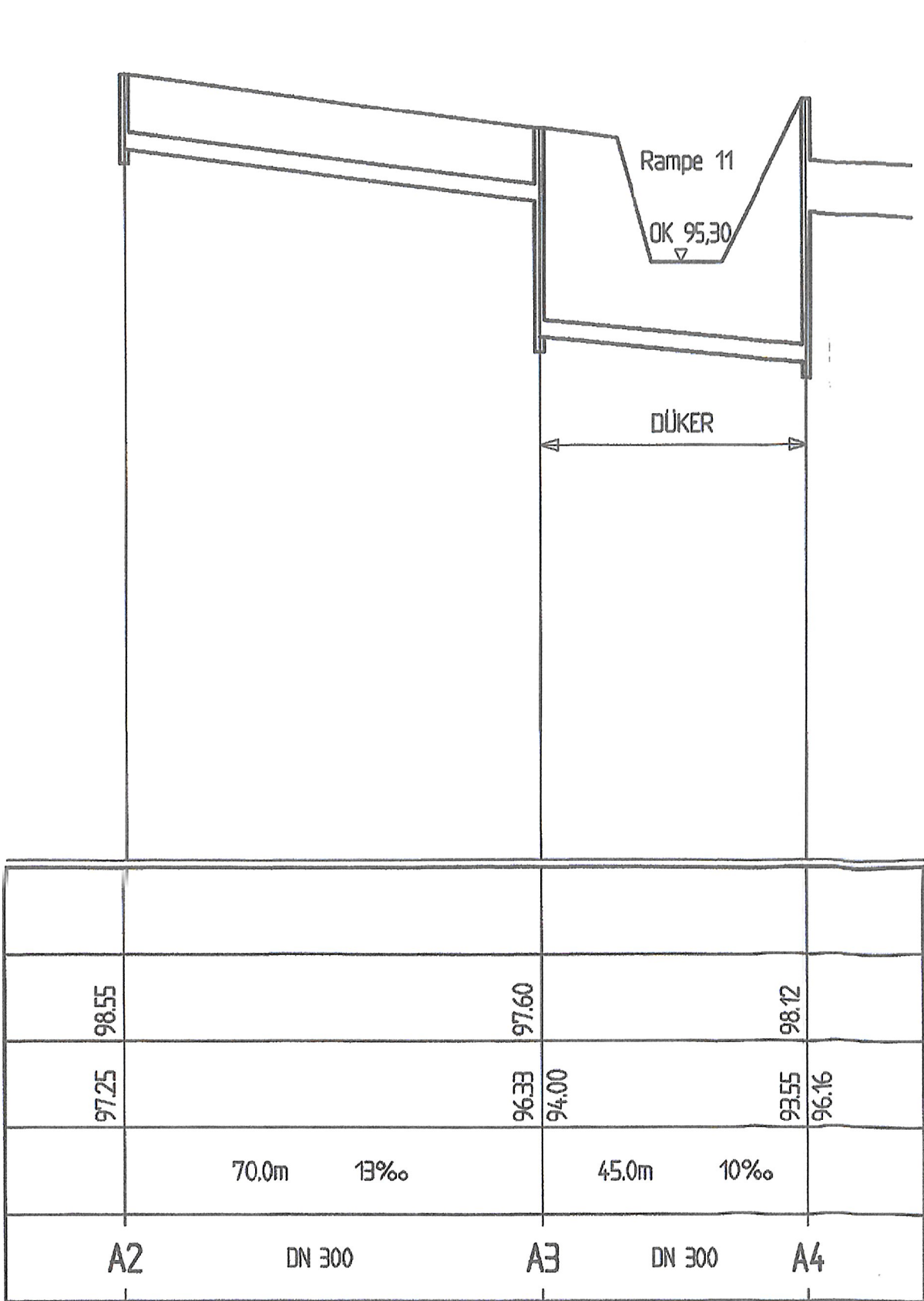
LÄNGENSCHNITT: SAMMLER A (A2-A4) MASSTAB: 1:1000/1:100
