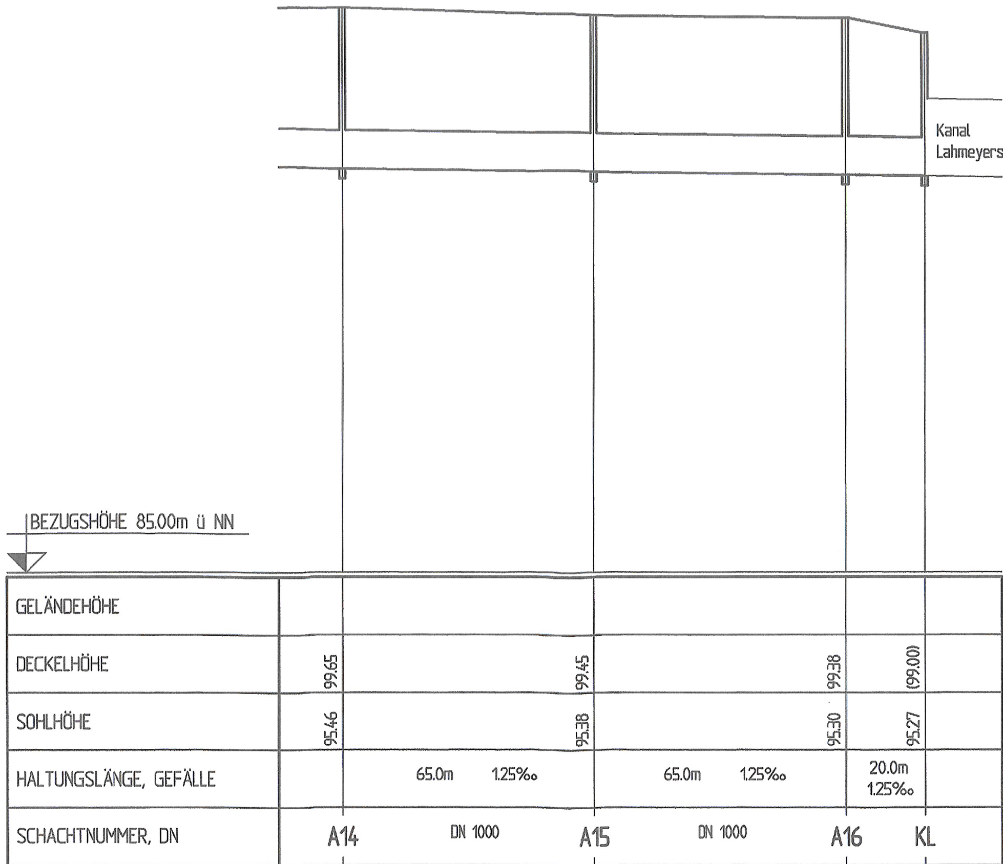
LÄNGENSCHNITT: SAMMLER R / A - ANSCHLUSS LAHMEYERSTRASSE MASSTAB: 1:1000/1:100
