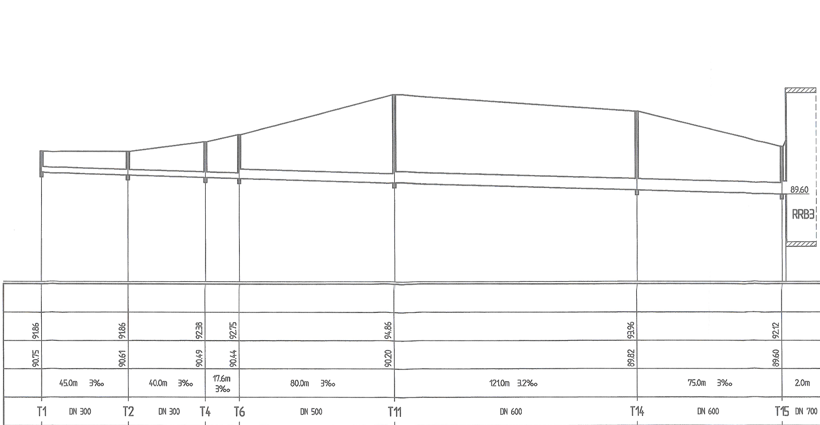
LÄNGENSCHNITT: SAMMLER T-TUNNEL MASSTAB: 1:1000/1:100
