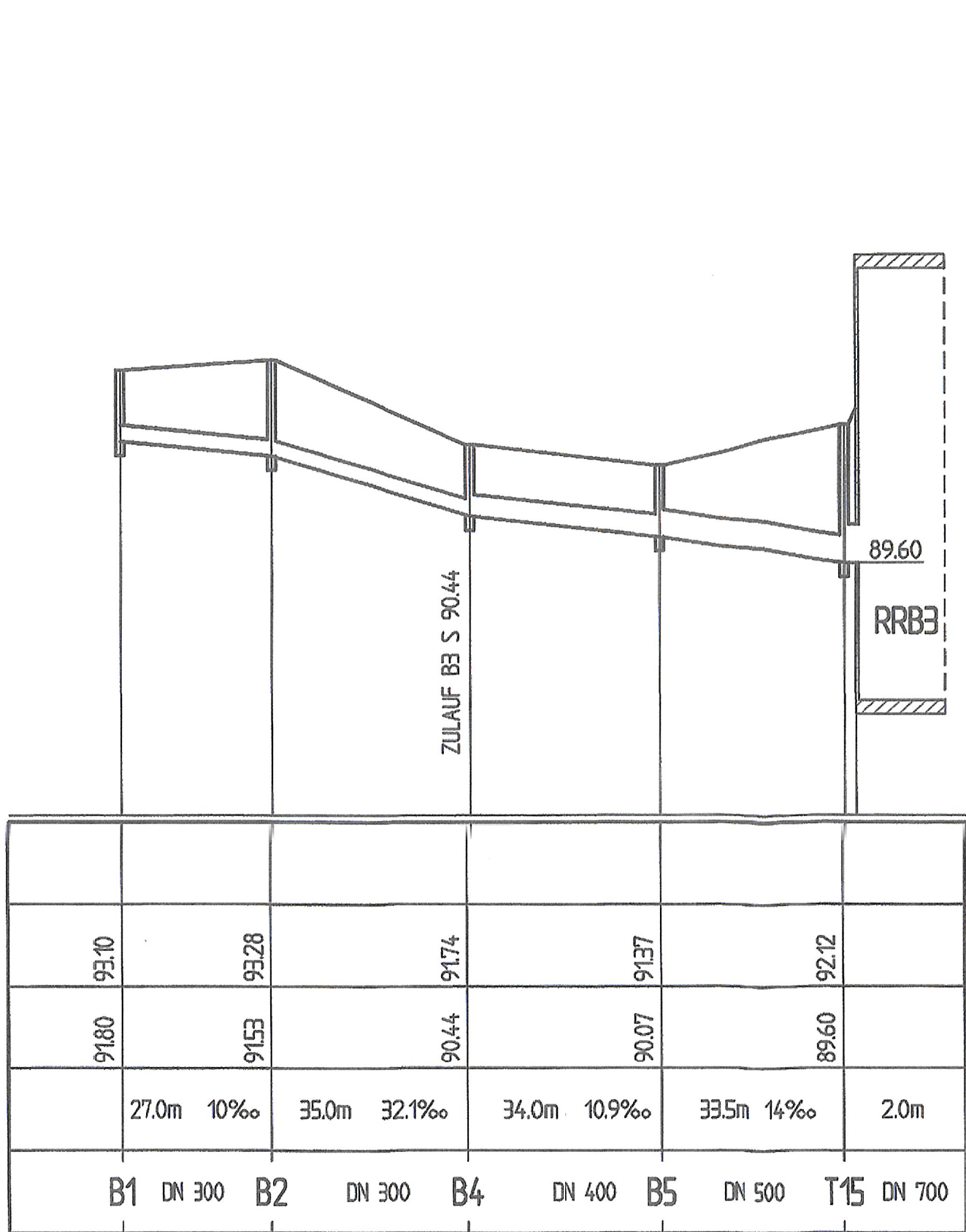
LÄNGENSCHNITT: SAMMLER B-RRB 3 MASSTAB: 1:1000/1:100
