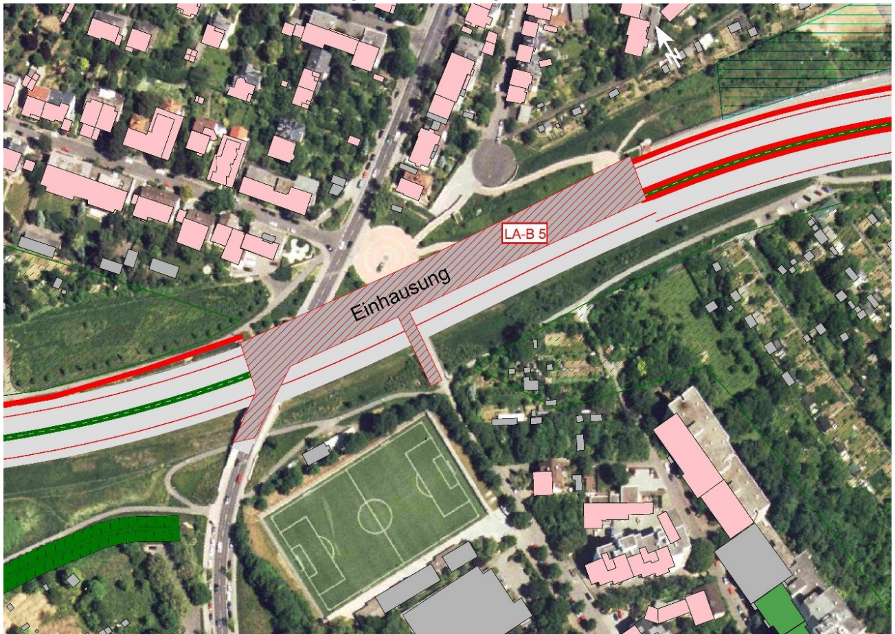
Abbildung 5 Galeriebauwerk im Bereich Seckbach [2]
