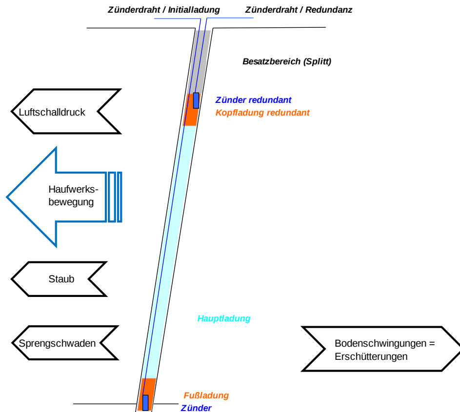
Abbildung 3 Schematische Darstellung der Emissionswirkungen einer Großbohrlochsprengung.
