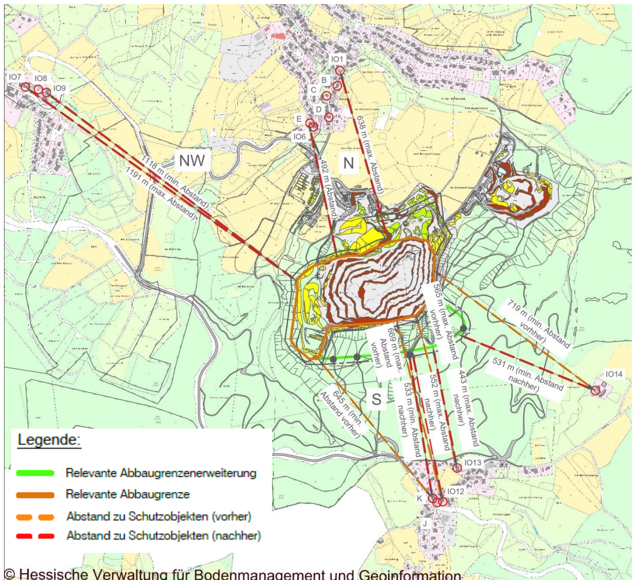
Abbildung 4 Genehmigter Abbau und Erweiterungsflächen mit den Immissionsorten (IO). Die Entfernungen zur Abbaugrenze bisher / zukünftig werden u.a. in nachfolgender Tabelle 2 angegeben. (Quelle: SST Prof. Dr.-Ing. Stoll & Partner Ingenieurgesellschaft mbH)
