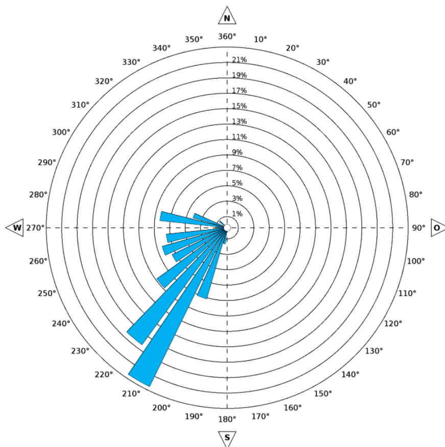
Abb. 6-4: Häufigkeitsverteilung der Windrichtung bei hohen Windgeschwindigkeit \geq 10.5 m/s der standortbezogenen meteorologischen Daten im Zeitraum 1995 bis 2012.
