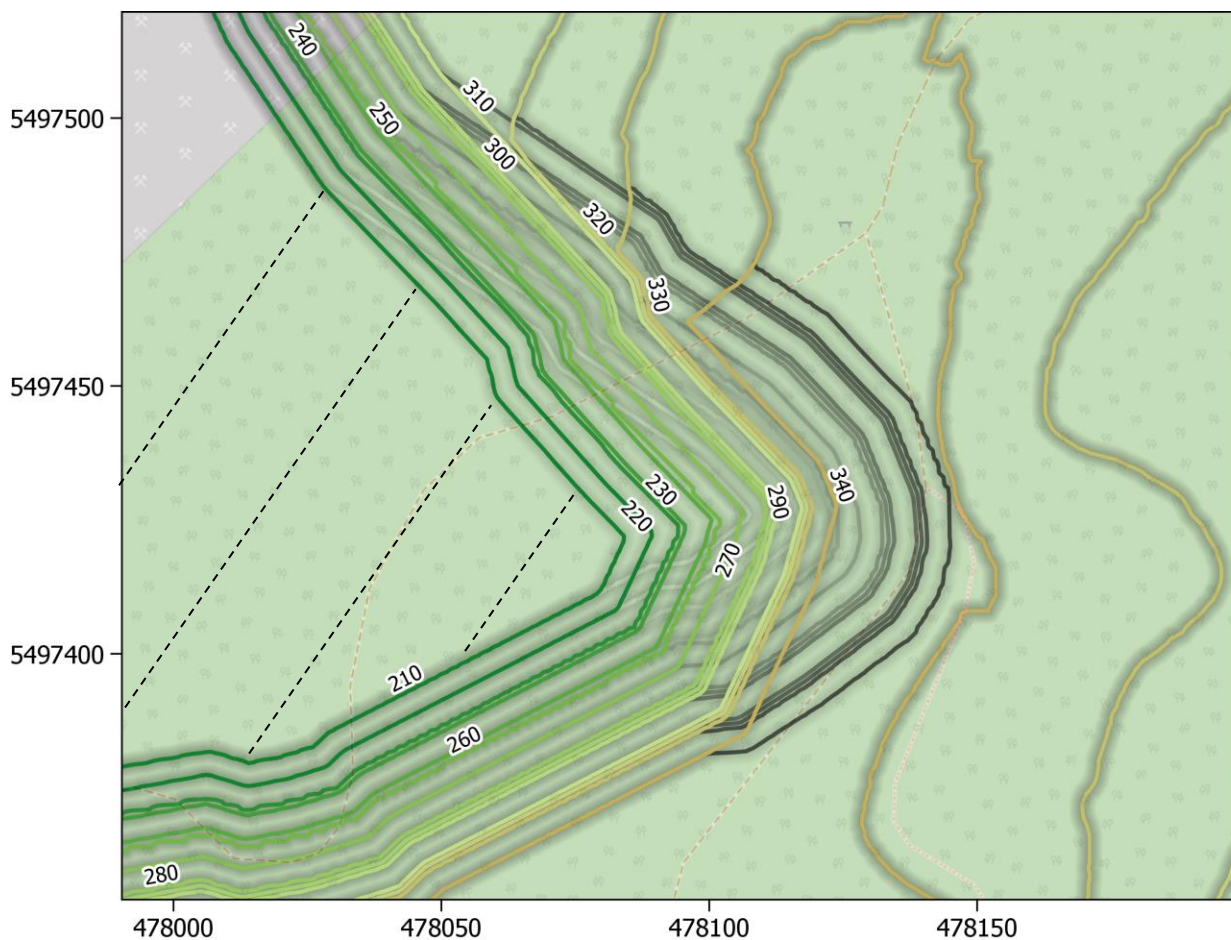
Abb. 4-3: Geländestruktur nach dem vollständigen Abbau (Isolinien mit Angabe Höhe über NN) an der östlichen Erweiterungskante für den Vorschlag des Forstamts (farbig) und für den vom Planungsbüro vorgesehenen Planfall (grau) (Kartengrundlage © OpenStreetMap-Mitwirkende).
