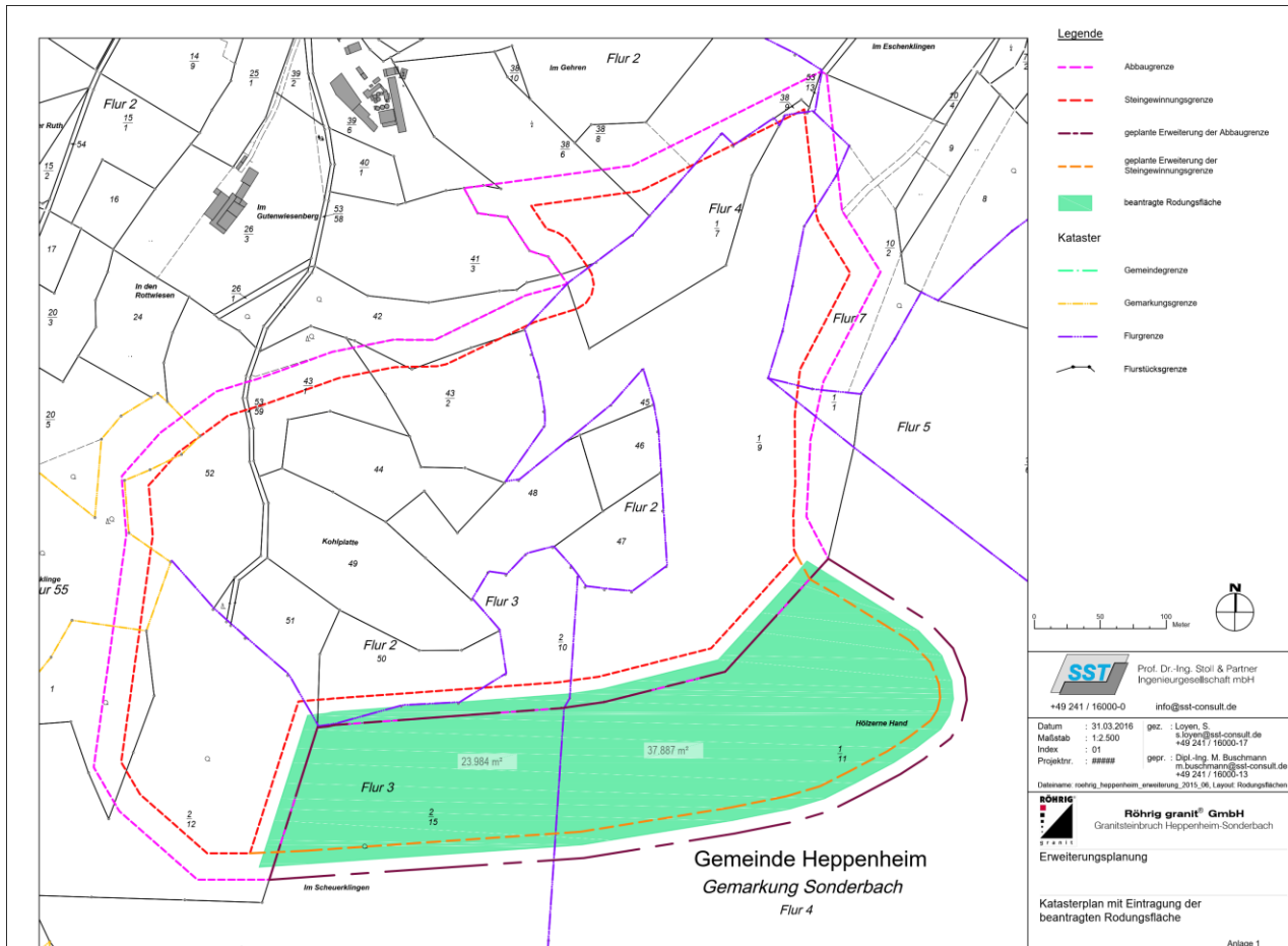
Abb. 4-1: Genehmigte (Magenta) und geplante Abbaugrenze (Violett) im Steinbruch Sonderbach (Stand 31.03.2016).
