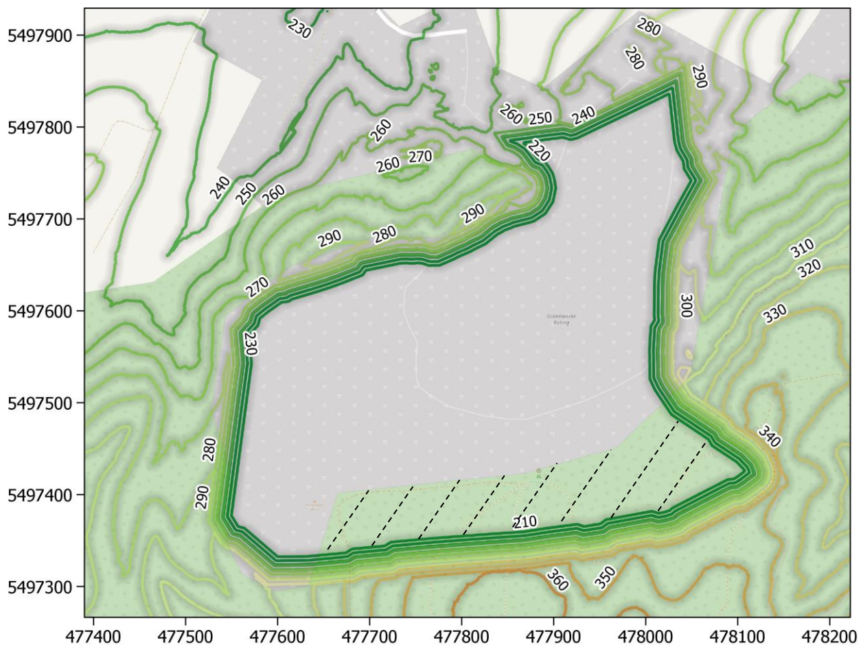
Abb. 4-2: Geländestruktur nach dem vollständigen geplanten Abbau (Isolinien mit Angabe Höhe über NN). Der im Erweiterungsbereich gerodete Wald ist schraffiert (Kartengrundlage © OpenStreetMap-Mitwirkende).
