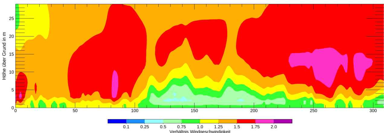
Abb. 6-6: Verhältnis der maximalen Windgeschwindigkeit in den unteren 30 m Höhe über Grund im Bereich der Abbaukante im Planfall (Lage siehe Abb. 5-3) zur ungestörten Anströmung.
