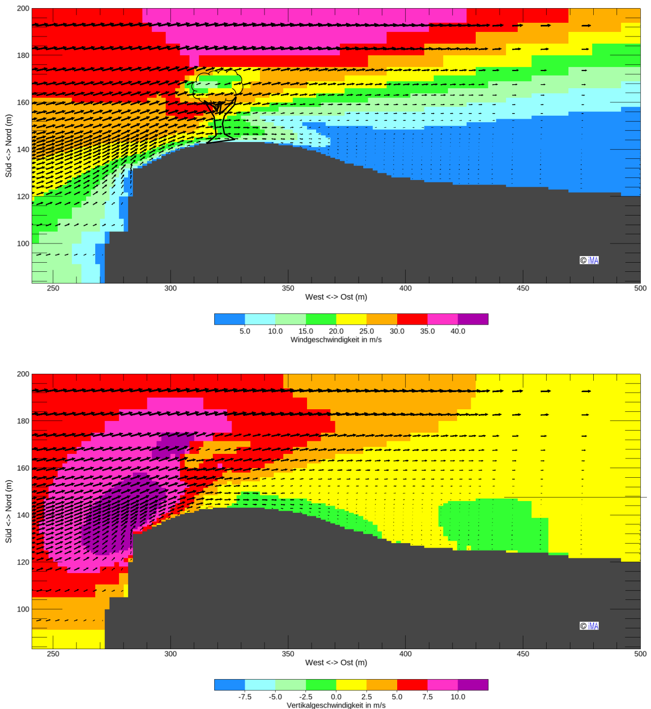
Abb. 1: Vertikalschnitt durch das Windfeld mit der berechneten mittleren horizontalen Windgeschwindigkeit (oben) und der Vertikalgeschwindigkeit (unten) bei einer Anströmrichtung von 260°. Oben skizziert ein Baum. In grau das unterliegende Gelände. Die Lage des Schnittes ist in Abb. 6-1 des Berichts dargestellt.
