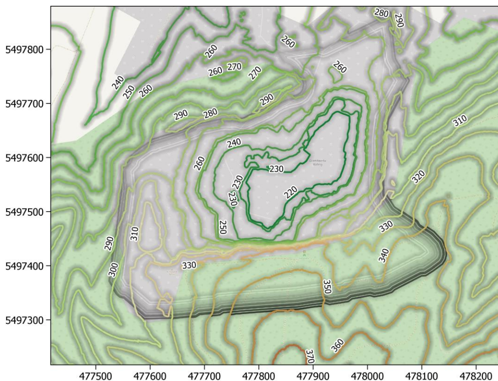
Abb. 3-2: Aktuelles Gelände (farbige Isolinien mit Angabe Höhe über NN), zukünftige Geländehöhen (graue Isolinien) und Nutzungsstruktur in der Umgebung des Steinbruchs (Kartengrundlage © OpenStreetMap-Mitwirkende).
