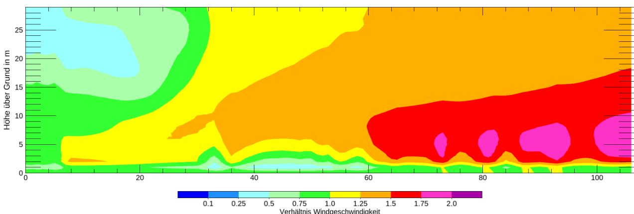
Abb. 6-8: Verhältnis der maximalen Windgeschwindigkeit in den unteren 30 m Höhe über Grund im Bereich der Abbaukante im Ist-Zustand (Lage siehe Abb. 5-3) zur ungestörten Anströmung.
