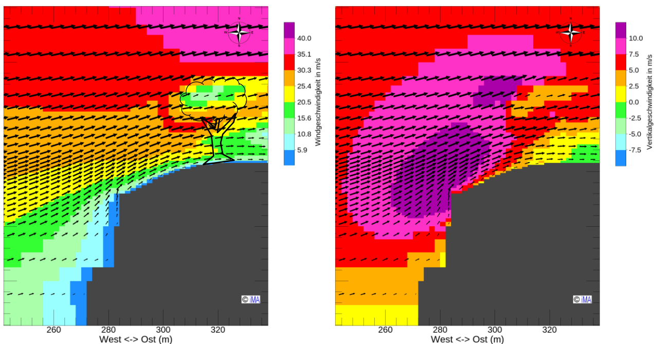
Abb. 6-2: Vertikalschnitt durch das Windfeld mit der berechneten mittleren horizontalen Windgeschwindigkeit (links) und der Vertikalgeschwindigkeit (rechts) bei einer Anströmrichtung von 260°. Links skizziert ein Baum. In grau das unterliegende Gelände. Die Lage des Schnittes ist in Abb. 6-1 dargestellt.
