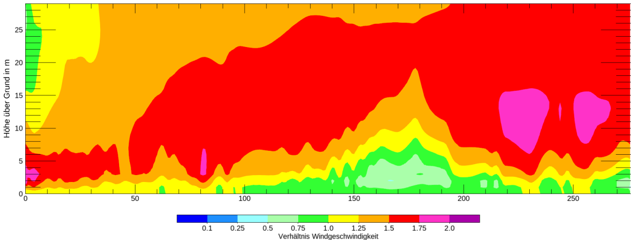
Abb. 6-7: Verhältnis der maximalen Windgeschwindigkeit in den unteren 30 m Höhe über Grund im Bereich der Abbaukante im Vorschlag des Forstamts (Lage siehe Abb. 5-3) zur ungestörten Anströmung.
