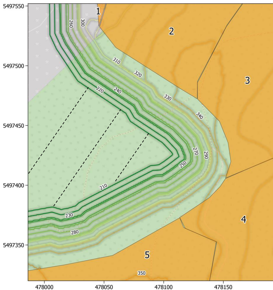
Abb. 5-1: Berücksichtigter Waldbestand nach Angaben des Auftraggebers (orange Flächen) in der Umgebung der östlichen Abbruchkante (Kartengrundlage © OpenStreetMap-Mitwirkende).
