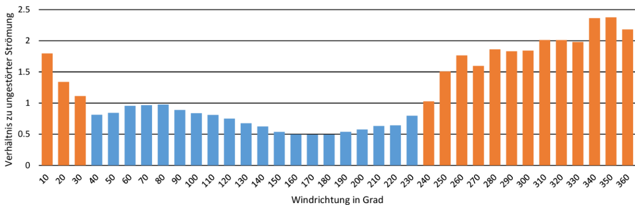
Abb. 6-3: Verhältnis der maximalen Windgeschwindigkeit in 10 m Höhe über Grund im Bereich der Abbaukante (Lage siehe Abb. 5-3) zur ungestörten Anströmung. Werte kleiner 1 (also niedriger als im ungestörten Fall) sind blau, Werte größer 1 orange eingefärbt.
