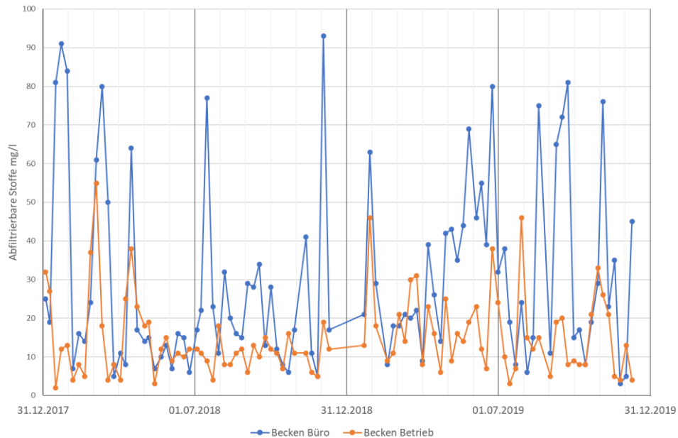
Abbildung 6 Verlauf der Konzentration an abfiltrierbaren Stoffen an der Abläufen 2018-2019, Datenquelle: Eigenüberwachung Fa. RÖHRIGgranit GmbH
