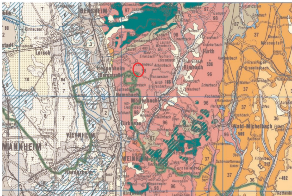
Bild 3.1: Ausschnitt aus der Geologischen Übersichtskarte von Hessen (siehe Unterlage [U02])
