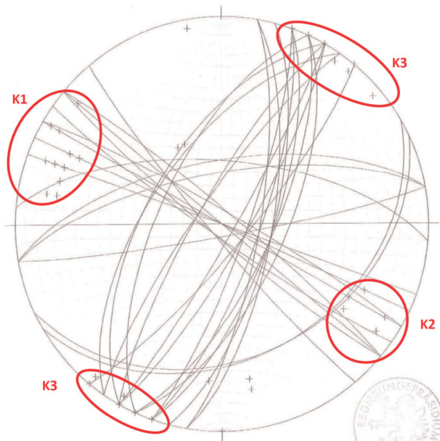
Bild 5.1: Raumstellung der Trennflächen gemäß Gefügaufnahme der Töniges GmbH (aus Unterlage [U09])
