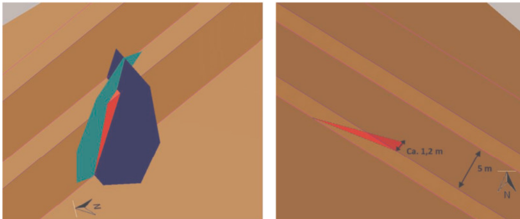
Bild 5.5: Ostwand - maßgebender Felskeil II (rot) – links: Schrägansicht Blickrichtung Südosten, rechts: Draufsicht (gewählte Trennfläche K2 (blau, Einfallrichtung/Einfallwinkel = 310^{\circ}/65^{\circ} ), gewählte Trennfläche K3 (türkis, Einfallrichtung/Einfallwinkel = 195^{\circ}/90^{\circ} ))
