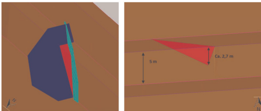
Bild 5.2: Südwand - maßgebender Felskeil I (rot) – links: Schrägansicht Blickrichtung Südosten, rechts: Draufsicht (gewählte Trennfläche K2 (blau, Einfallrichtung/Einfallwinkel = 290^\circ/65^\circ ), gewählte Trennfläche K3 (türkis, Einfallrichtung/Einfallwinkel = 25^\circ/90^\circ ))
