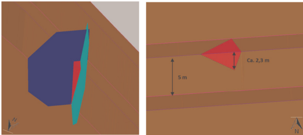
Bild 5.3: Südwall - maßgebender Felskeil II (rot) – links: Schrägansicht Blickrichtung Südosten, rechts: Draufsicht (gewählte Trennfläche K2 (blau, Einfallrichtung/Einfallwinkel = 290^{\circ}/85^{\circ} ), gewählte Trennfläche K3 (türkis, Einfallrichtung/Einfallwinkel = 25^{\circ}/80^{\circ} ))
