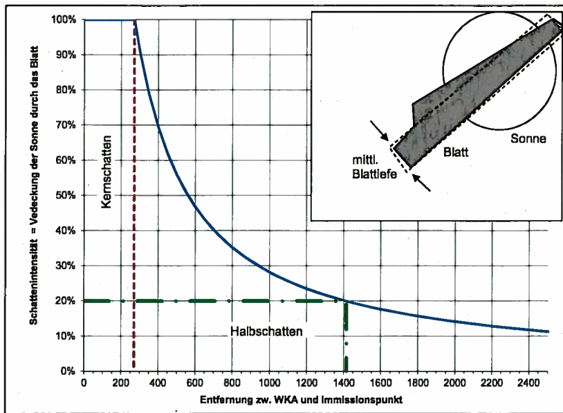
Intensität des Schattens in Abhängigkeit der Entfernung bei einer Fuhränder FL MD 77 mit 85m Nabenhöhe und 2,08m mittlerer Blatttiefe
