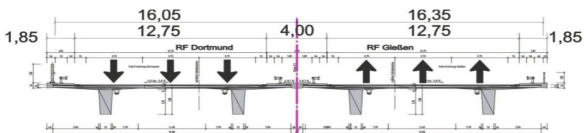
Abb. 2: Bestandsquerschnitt Talbrücke
