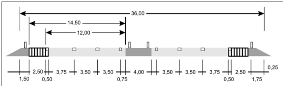
Abb. 6: geplanter Regelquerschnitt RQ 36
