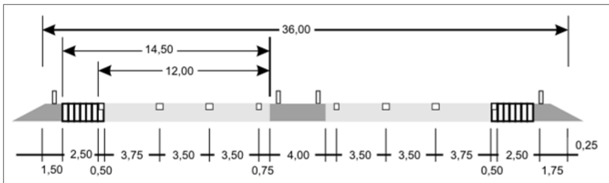
Abb. 4: geplanter Streckenregelquerschnitt RQ 36
