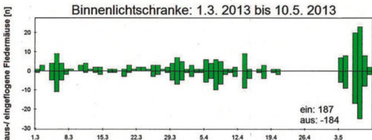
Abbildung 6: Fledermausaktivität am Fotofallenstandort „Kalkabbaustollen“ auf Basis artbestimmter Fotos ausfliegender Fledermäuse im Zeitraum 1.3.–10.05.2013 im eingangsfernen Gangsystem
