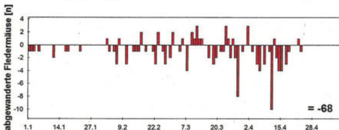
Abbildung 12: Abwanderungsverlauf überwinterter Fledermäuse aus dem Stollen „Rosengarten“ zwischen dem 1. Januar und 10. Mai 2013 auf der Basis von bilanzierten Lichtschrankenregistrierungen.
