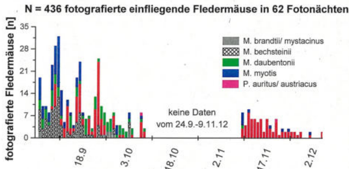
Abbildung 10: Fledermausaktivität am Fotofallenstandort „Rosengarten“ auf Basis artbestimmter Fotos einfliegender Fledermäuse im Zeitraum 14.9.–11.12.2012
