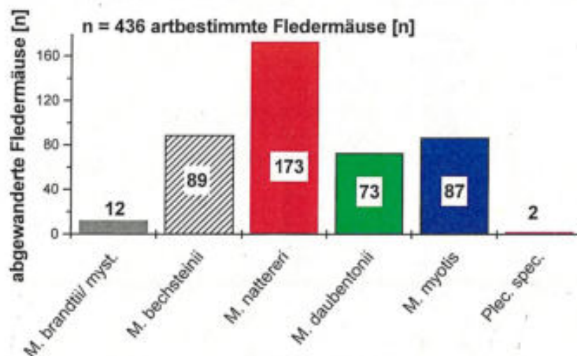
Abbildung 10: Fledermausaktivität am Fotofallenstandort „Rosengarten“ auf Basis artbestimmter Fotos einfliegender Fledermäuse im Zeitraum 14.9.–11.12.2012
