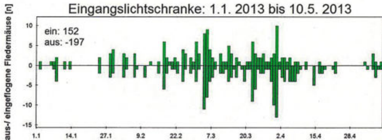
Abbildung 4: Fledermausaktivität an der Eingangslichtschanke zum „Kalkabbaustollen“ zwischen dem 1. Januar und 10. Mai 2013 auf der Basis von Lichtschankenregistrierungen
