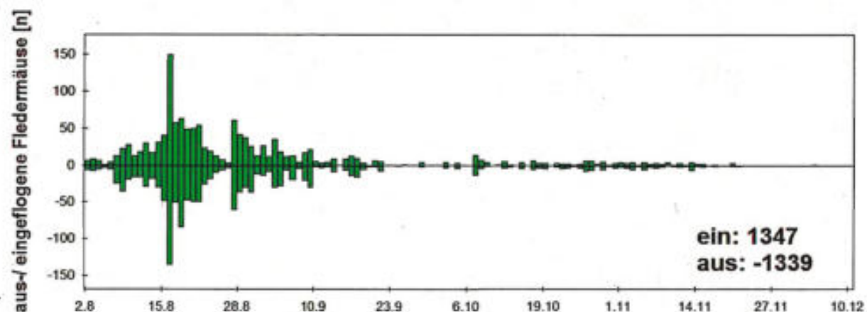
Abbildung 1: Fledermausaktivität am „Kalkabbaustollen“ zwischen dem 2. August und 11. Dezember 2012 auf der Basis von Lichtschrankenregistrierungen
