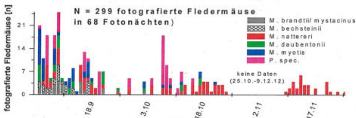
Abbildung 3: Fledermausaktivität am Fotofallenstandort „Kalkabbaustollen“ auf Basis artbestimmter Fotos einfliegender Fledermäuse im Zeitraum 14.9.–11.12.2012.
