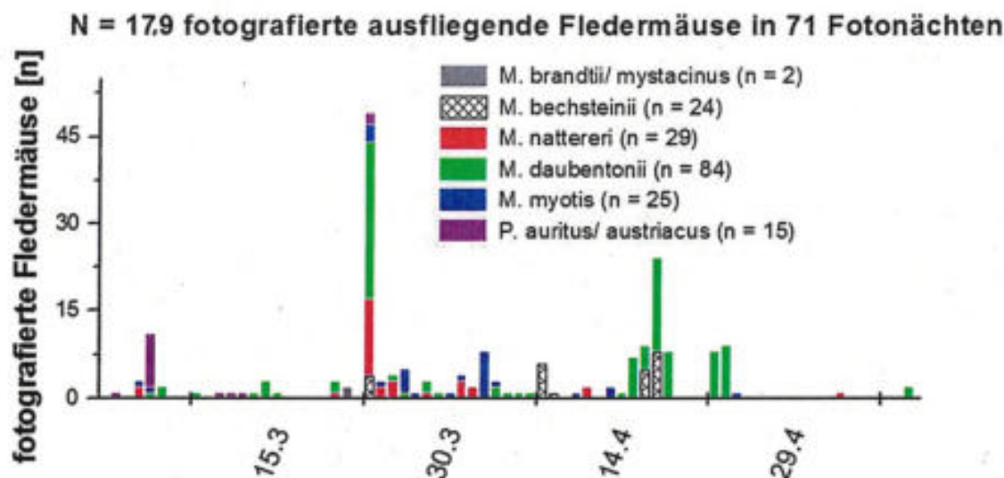
Abbildung 7: Aktivitätsverlauf auf Basis artbestimmter Fotos ausfliegender Fledermäuse am Fotofallenstandort „Kalkabbaustollen“ im Zeitraum 1.3.–10.05.2013
