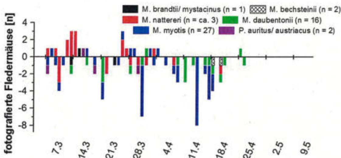
Abbildung 14: Abgewanderte Winterschläfer am Fotofallenstandort „Rosengarten“ auf Basis artbestimmter bilanzierter Fotos im Zeitraum 28.2.–10.05.2013
