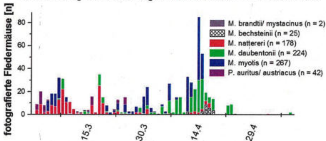
Abbildung 13: Fledermausaktivität am Fotofallenstandort „Rosengarten“ auf Basis artbestimmter Fotos ausfliegender Fledermäuse im Zeitraum 28.2.–10.05.2013
