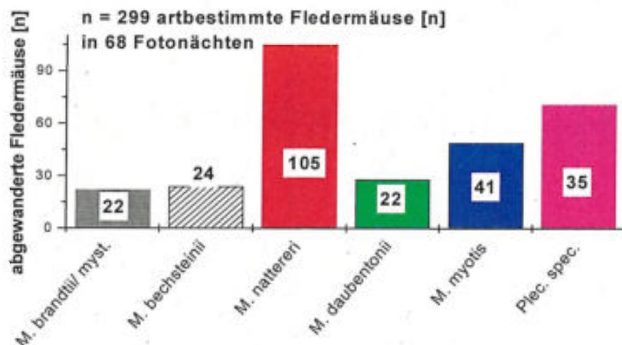
Abbildung 2: Nachweishäufigkeit der verschiedenen Fledermausarten am Fotofallenstandort „Kalkabbaustollen“ auf Basis artbestimmter Fotos einfliegender Fledermäuse im Zeitraum 14.9.–11.12.2012
