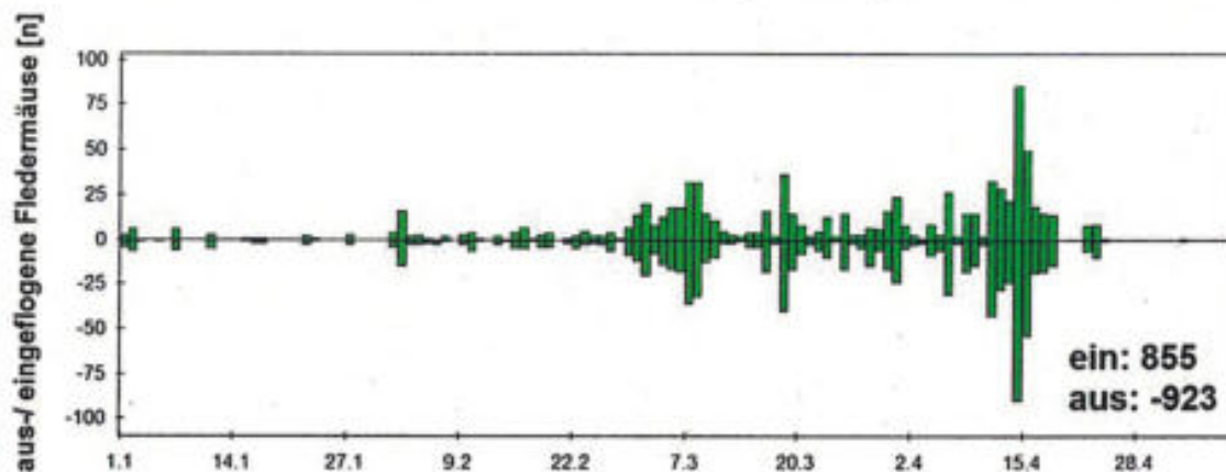
Abbildung 11: Fledermausaktivität am Stollen „Rosengarten“ zwischen dem 1. Januar und 10. Mai 2013 auf der Basis von Lichtschrankenregistrierungen
