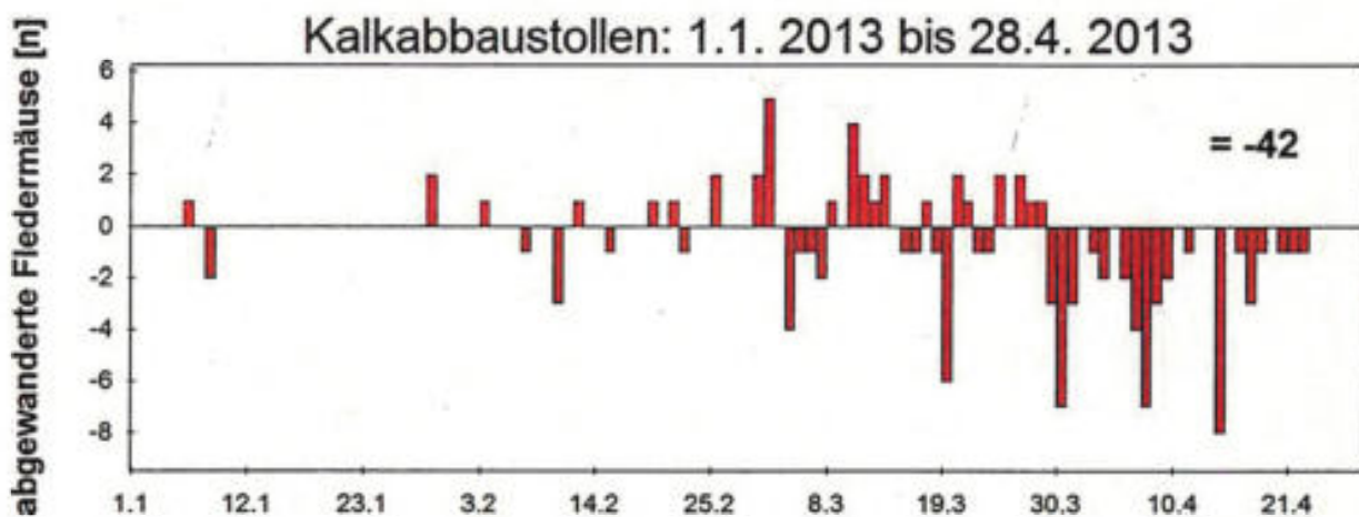
Abbildung 5: Abwanderungsverlauf überwinterter Fledermäuse aus dem „Kalkabbaustollen“ zwischen dem 1. Januar und 10. Mai 2013 auf der Basis von bilanzierten Lichtschankenregistrierungen
