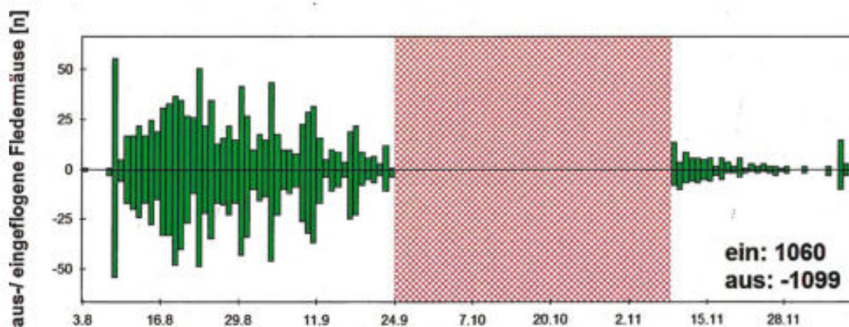
Abbildung 8: Fledermausaktivität am Stollen „Rosengarten“ zwischen dem 2. August und 11. Dezember 2012 auf der Basis von Lichtschrankenregistrierungen. Wegen eines Kabeldefektes liegen für den Zeitraum 24.9.-9.11.12 keine Daten vor.
