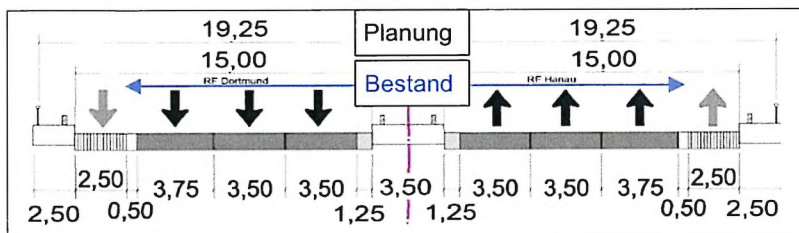
Abbildung 3: geplanter Brückenregelquerschnitt RQ 36 B
