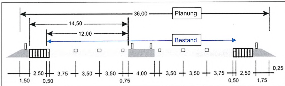
Abbildung 2: geplanter Streckenregelquerschnitt RQ 36
