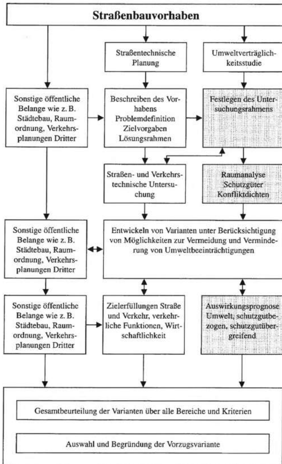
Abb. 1: Die UVS innerhalb der Straßenplanung – integrative Abfolge und Zuordnung wichtiger Untersuchungen (FGSV 2001)
