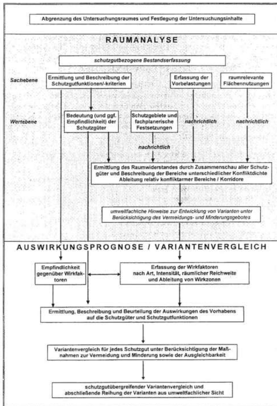
Abb. 2: Arbeitsschritte und Planungsablauf einer Umweltverträglichkeitsstudie (HLSV 2000)
