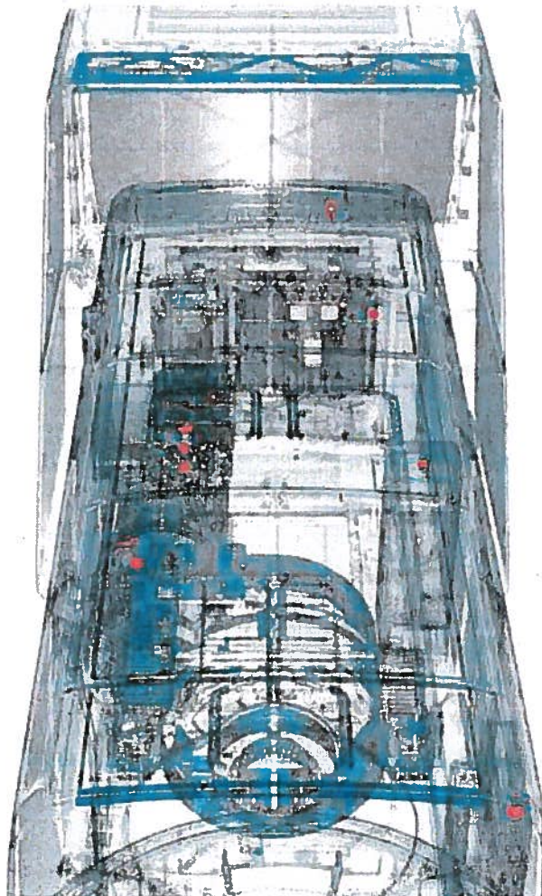
Abbildung 6-1: Rauchmeldeanlage (rot) im Maschinenhaus (2.0 MW, Mk 8 wird als Beispiel verwendet)
