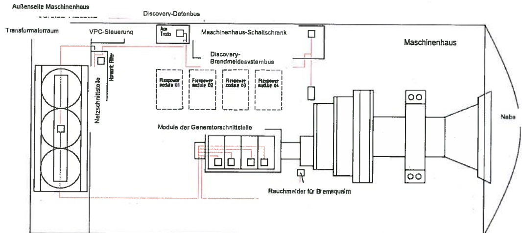
Abbildung 7-2: Beispiel für Systemaufbau in V112-3.0 MW
