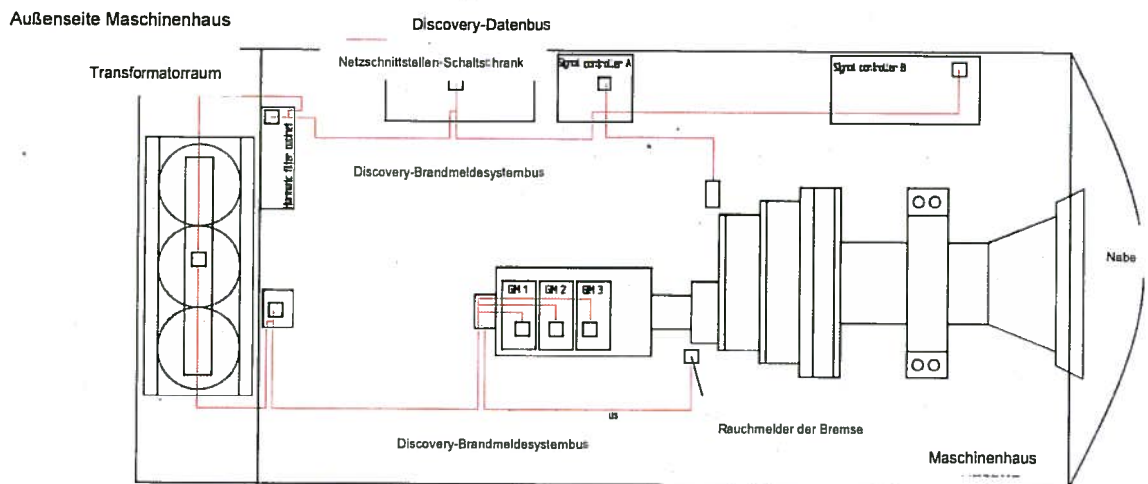
Abbildung 7-1: Beispiel für Systemaufbau in 2.0 MW, Mk 8
