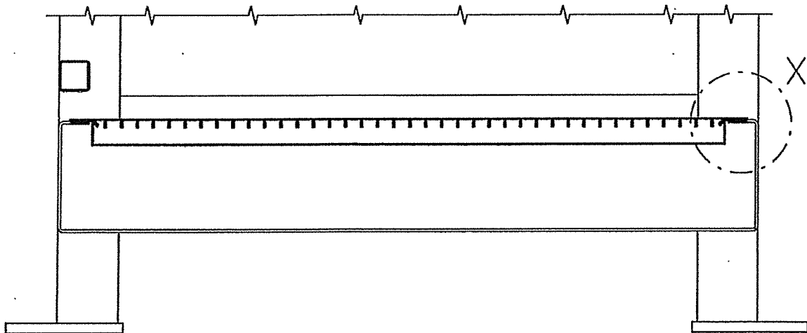
Einbaudetail Gitterroste
