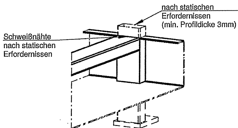
Anbindung Mittelrahmen
