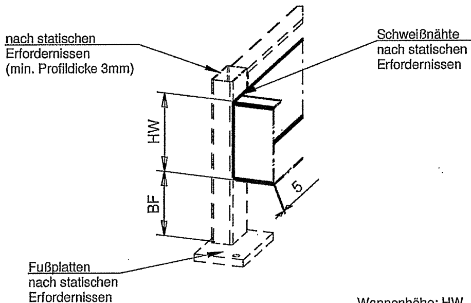
Anbindung Außenrahmen
