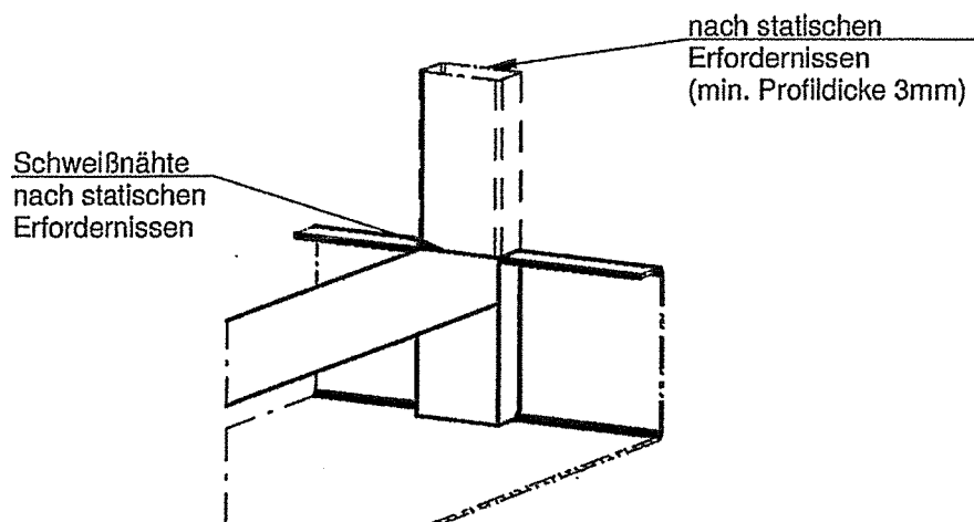
Anbindung Mittelrahmen
