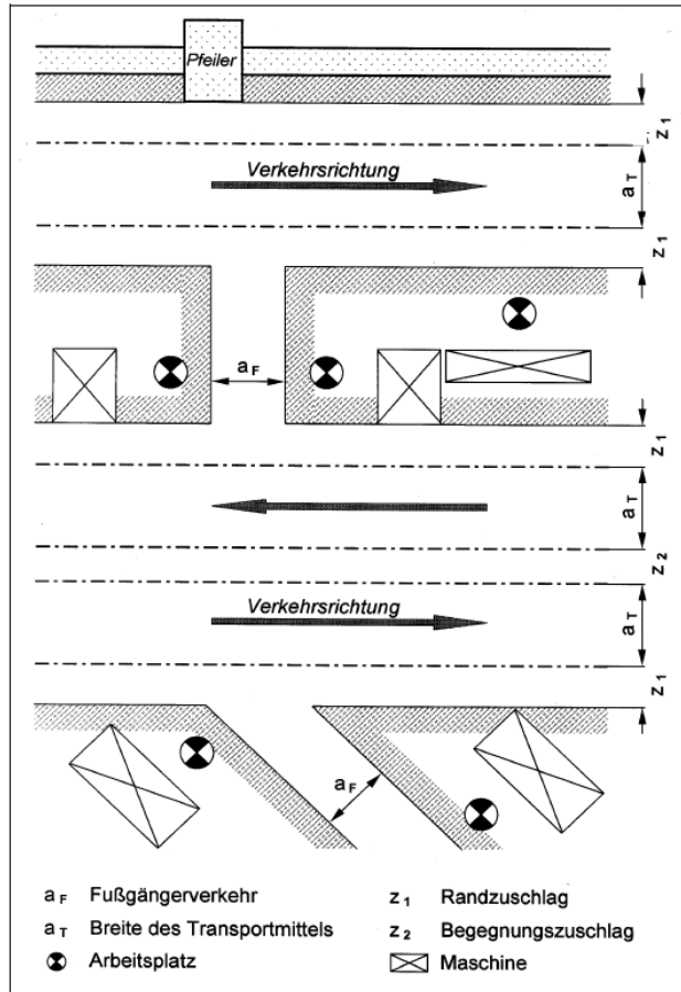
Abb. 3: Verkehrswegebreiten, Sicherheitszuschläge (siehe auch Tabellen 2 und 3)
