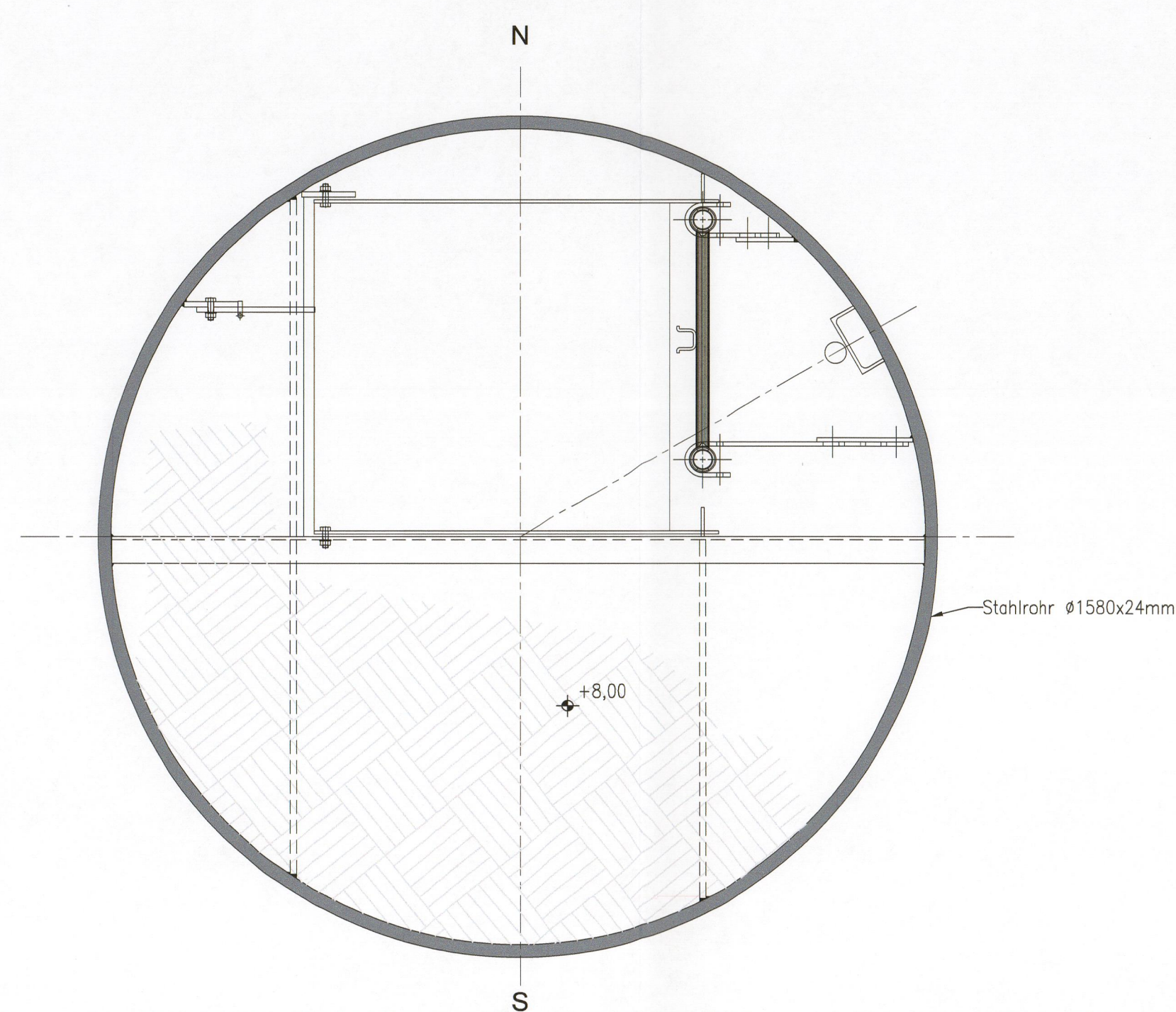
Schnitt A-A M. 1:10
