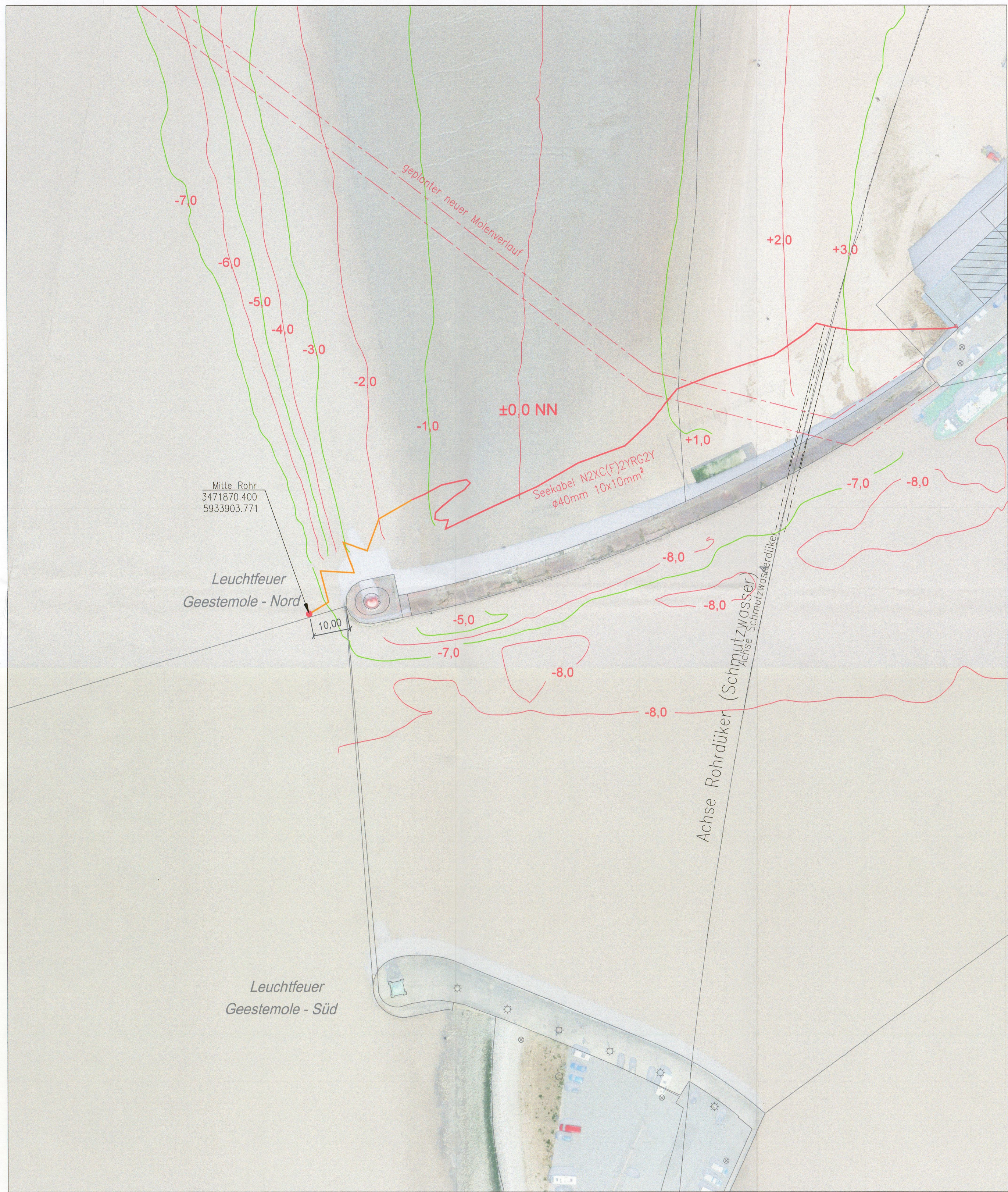
Lageplan M. 1:750
