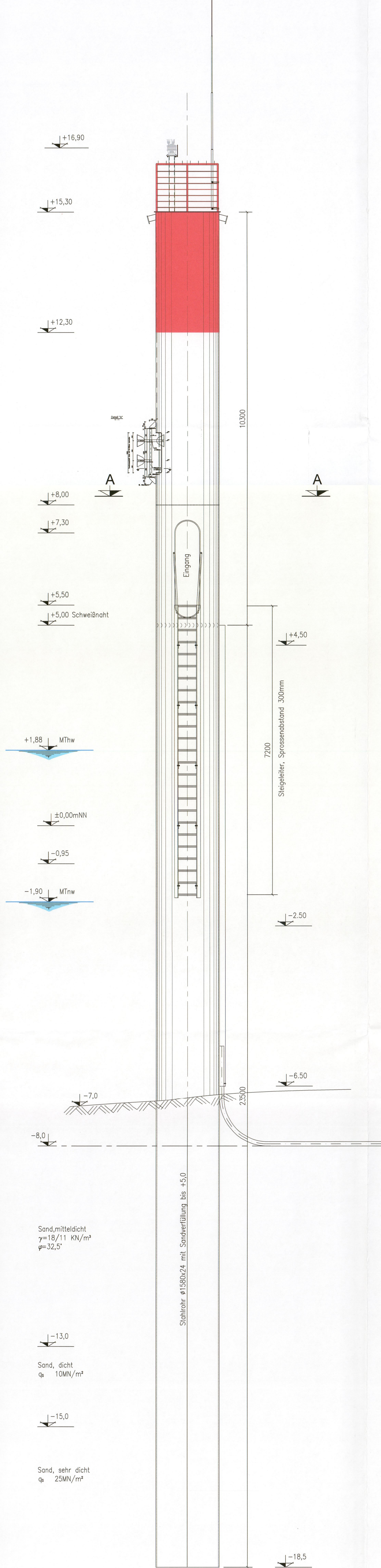
Südsansicht M. 1:50
