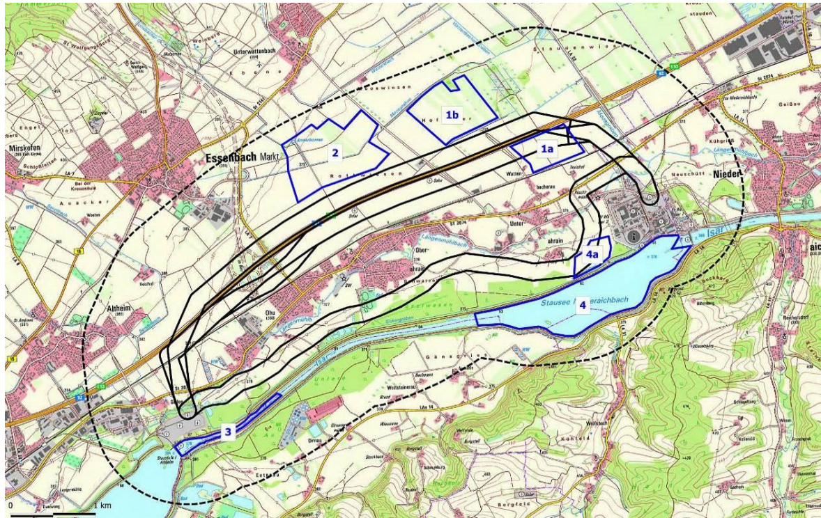
Abbildung 9: Lage der Rastgebiete 1 bis 4
