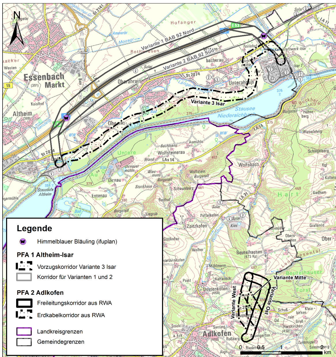
Abbildung 102: Nachweise Himmelblauer Bläuling gemäß eigenen Kartierungen 2022
