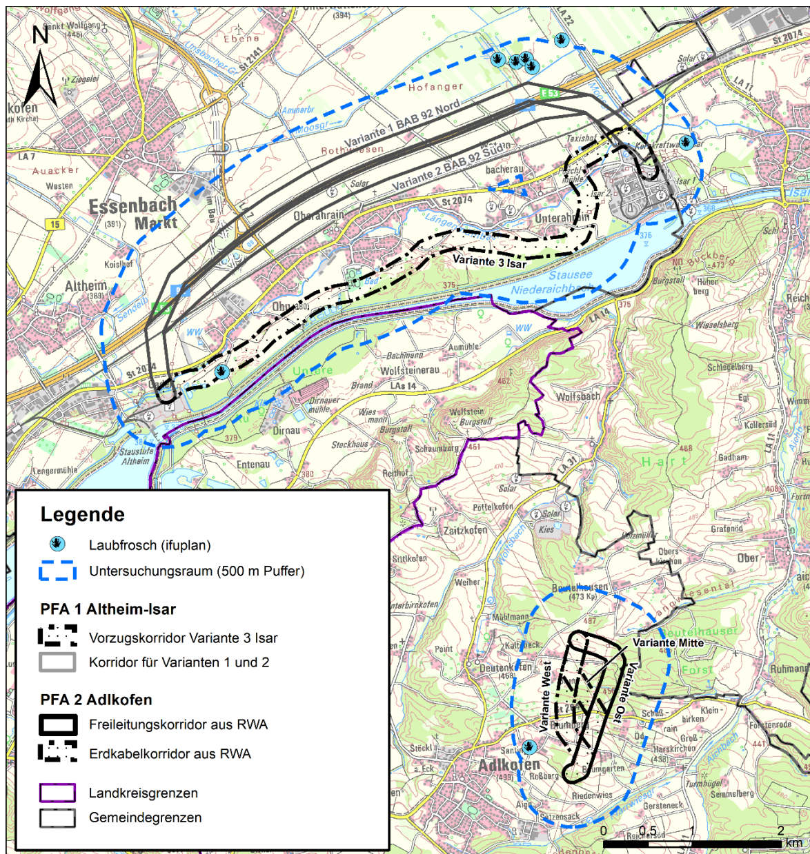
Abbildung 98: Nachweise Laubfrosch gemäß eigenen Kartierungen 2022
