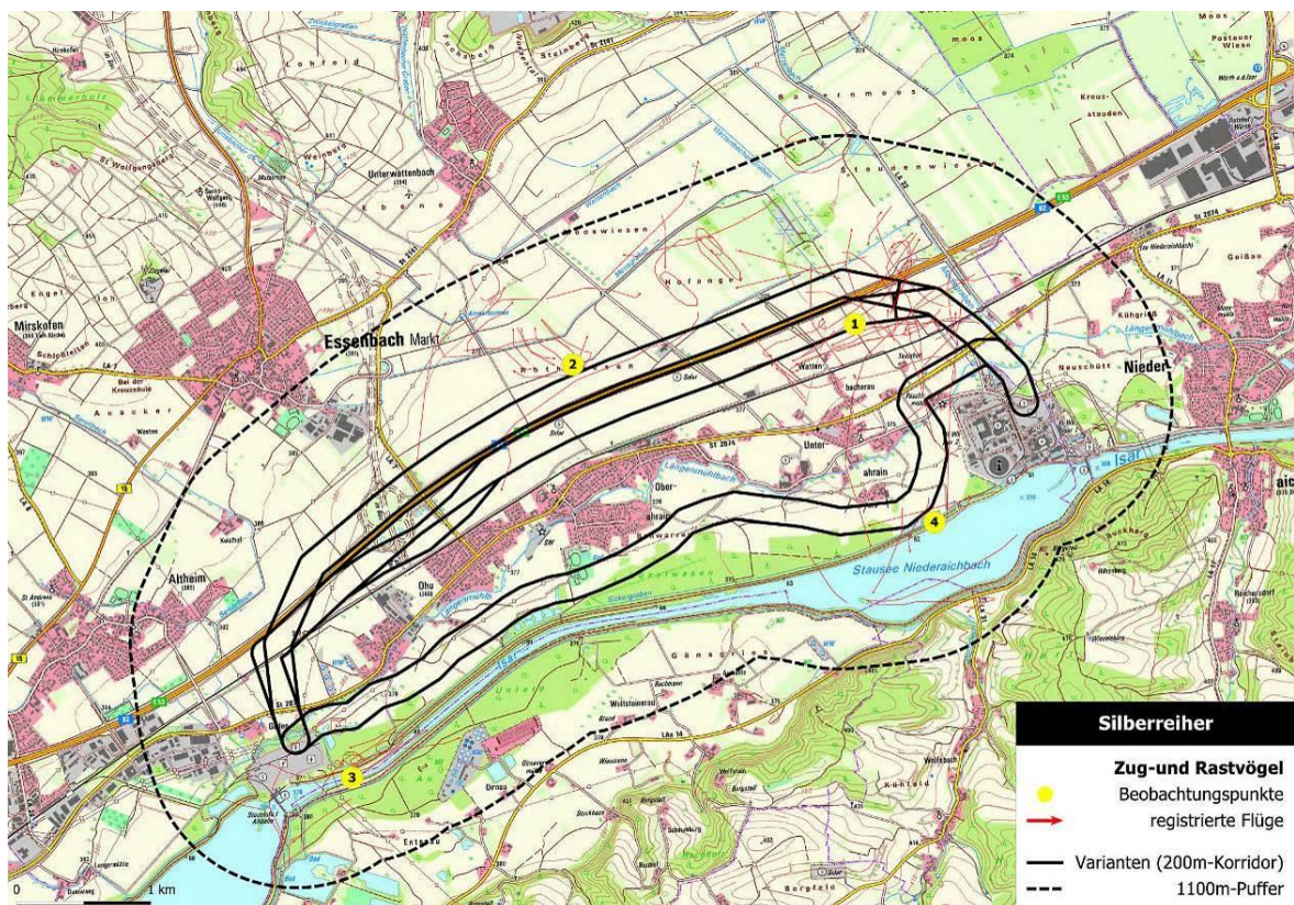
Abbildung 58: Flugrouten von Silberreiher
