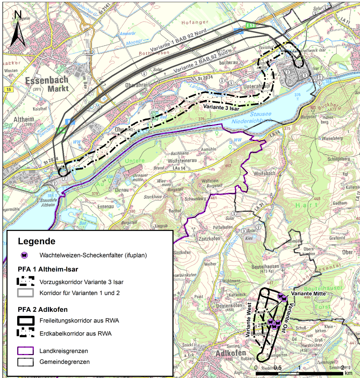
Abbildung 103: Nachweise Wachtelweizen-Scheckenfalter gemäß eigenen Kartierungen 2022
