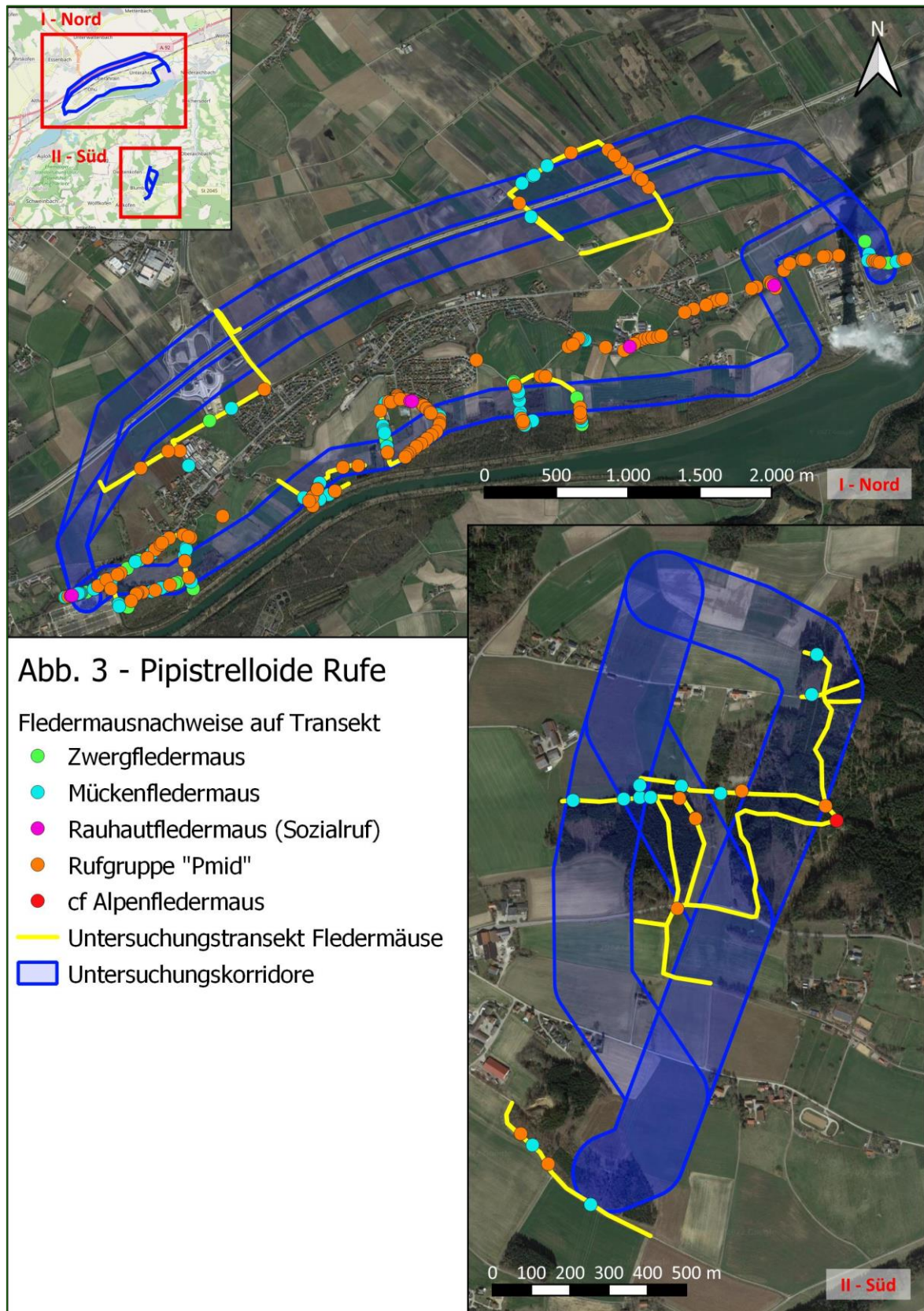
Abbildung 87: Pipistrelloide Rufe (Datengrundlage © 2022 GeoBasis-DE/BKG, GeoContent, Maxar Technologies)
