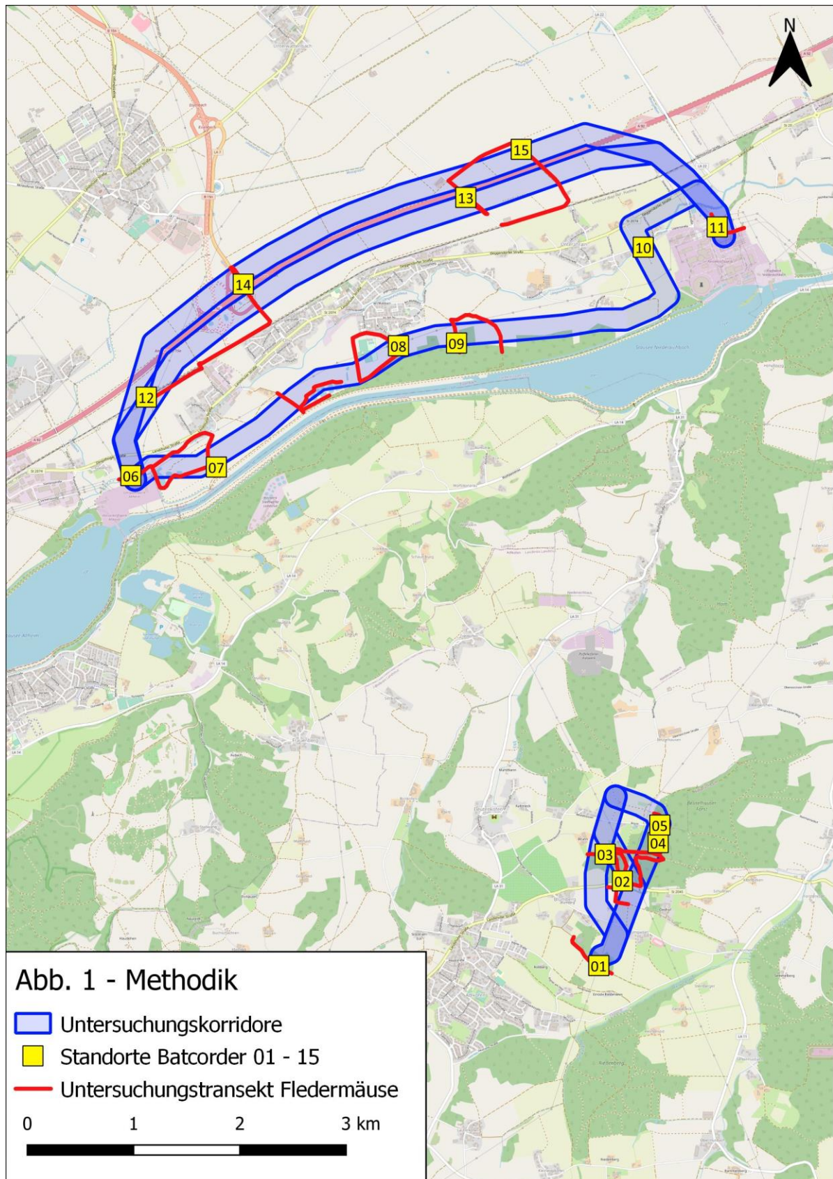
Abbildung 84: Untersuchungsraum Fledermäuse (Geobasisdaten: © OpenStreetMap (ODbL) & OpenStreetMap contributors)
