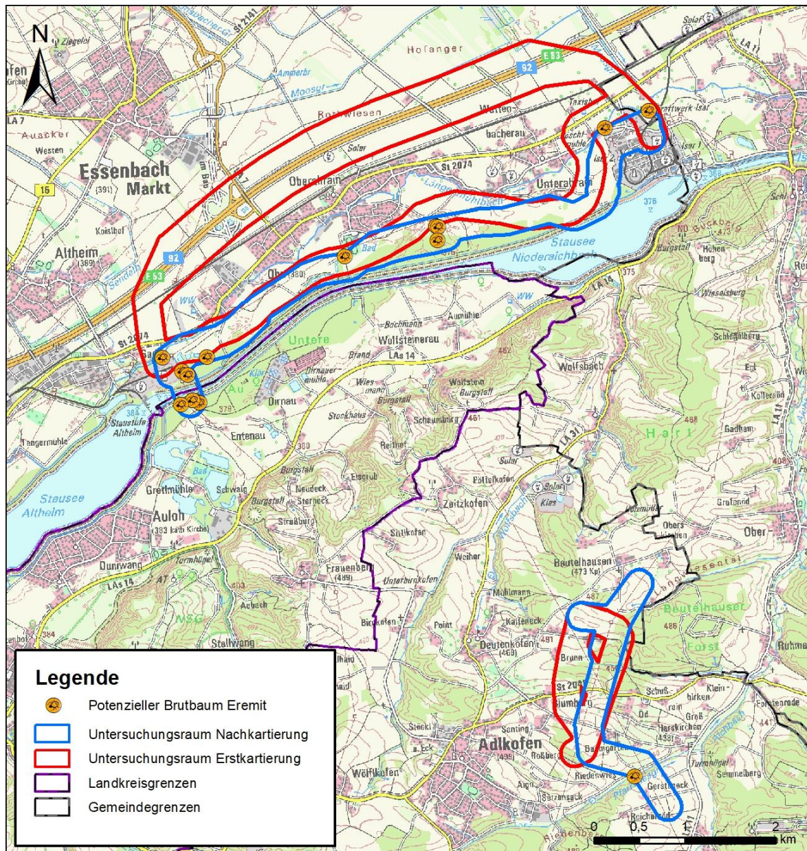
Abbildung 112: Potenzielle Brutbäume für den Eremit
