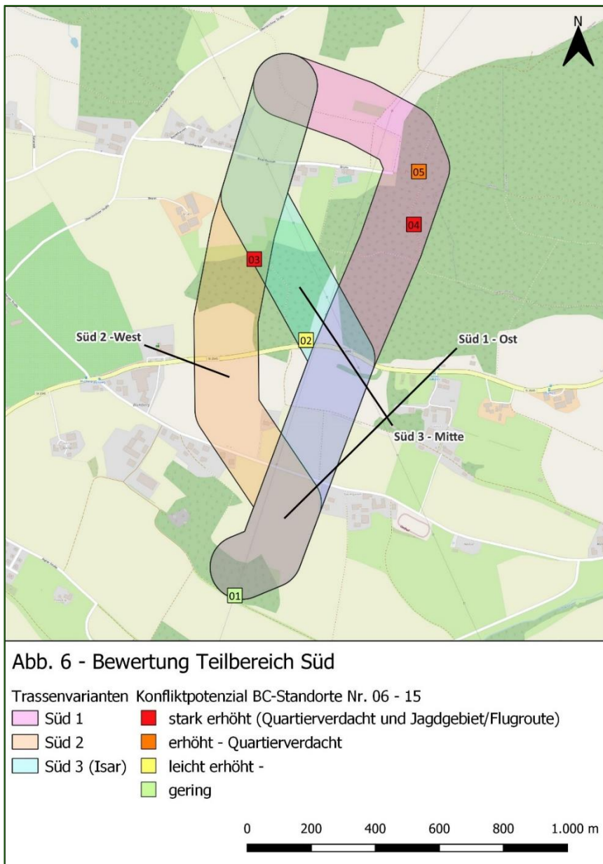
Abbildung 91: Bewertung Teilbereich Süd
