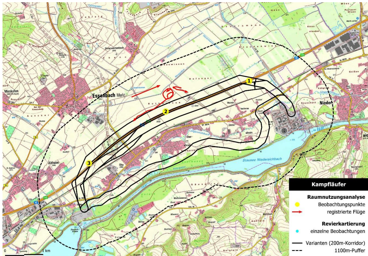
Abbildung 63: Räumliche Verteilung der Beobachtungen von Kampfläuffern
