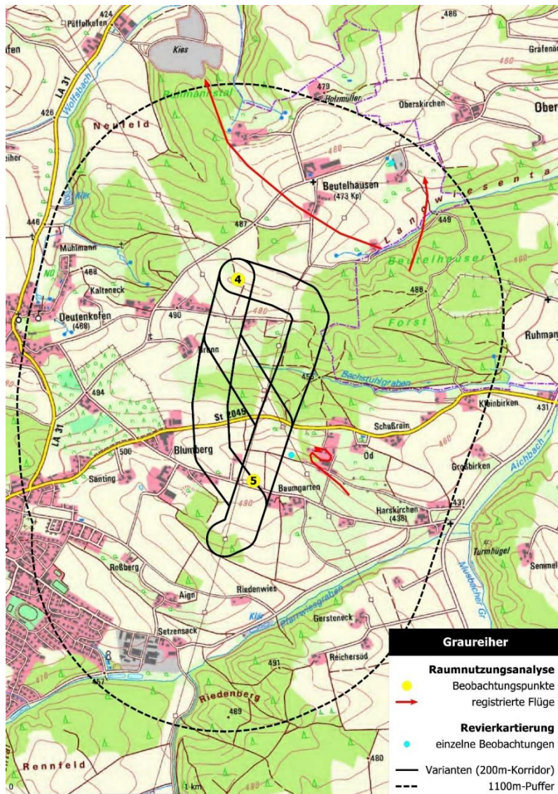
Abbildung 79: Räumliche Verteilung der Beobachtungen von Graureihern
