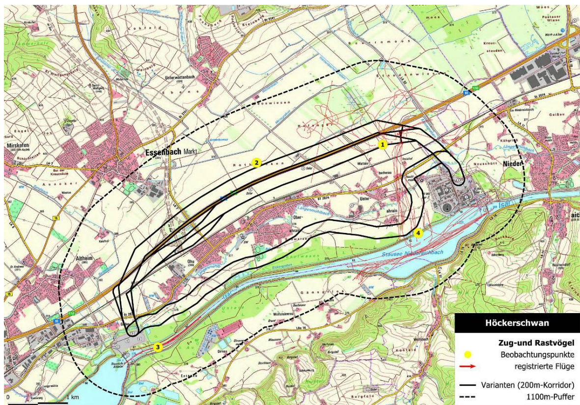
Abbildung 54: Flugrouten von Höckerschwänen
