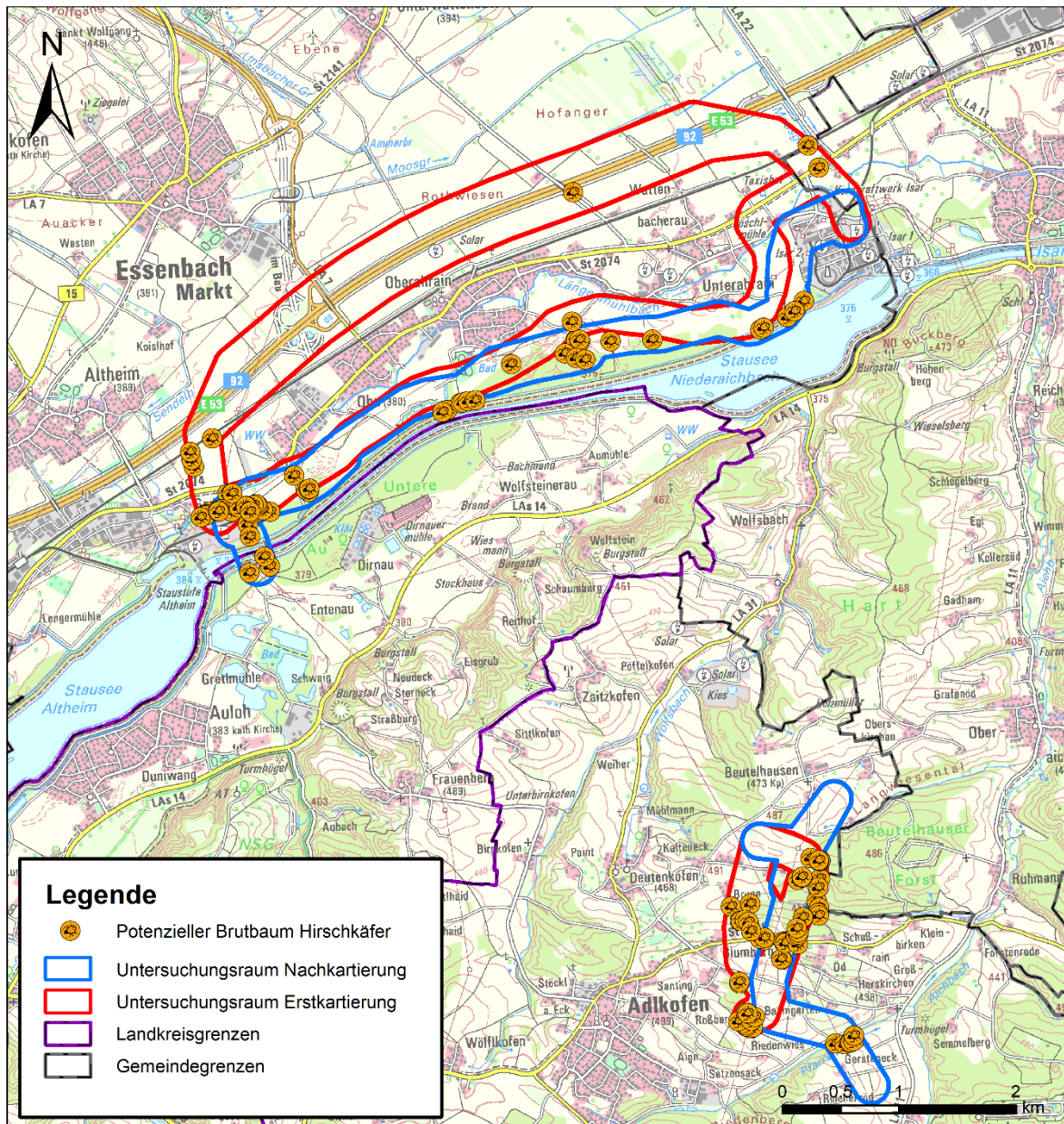
Abbildung 111: Potenzielle Soft- und Brutbäume für den Hirschkäfer
