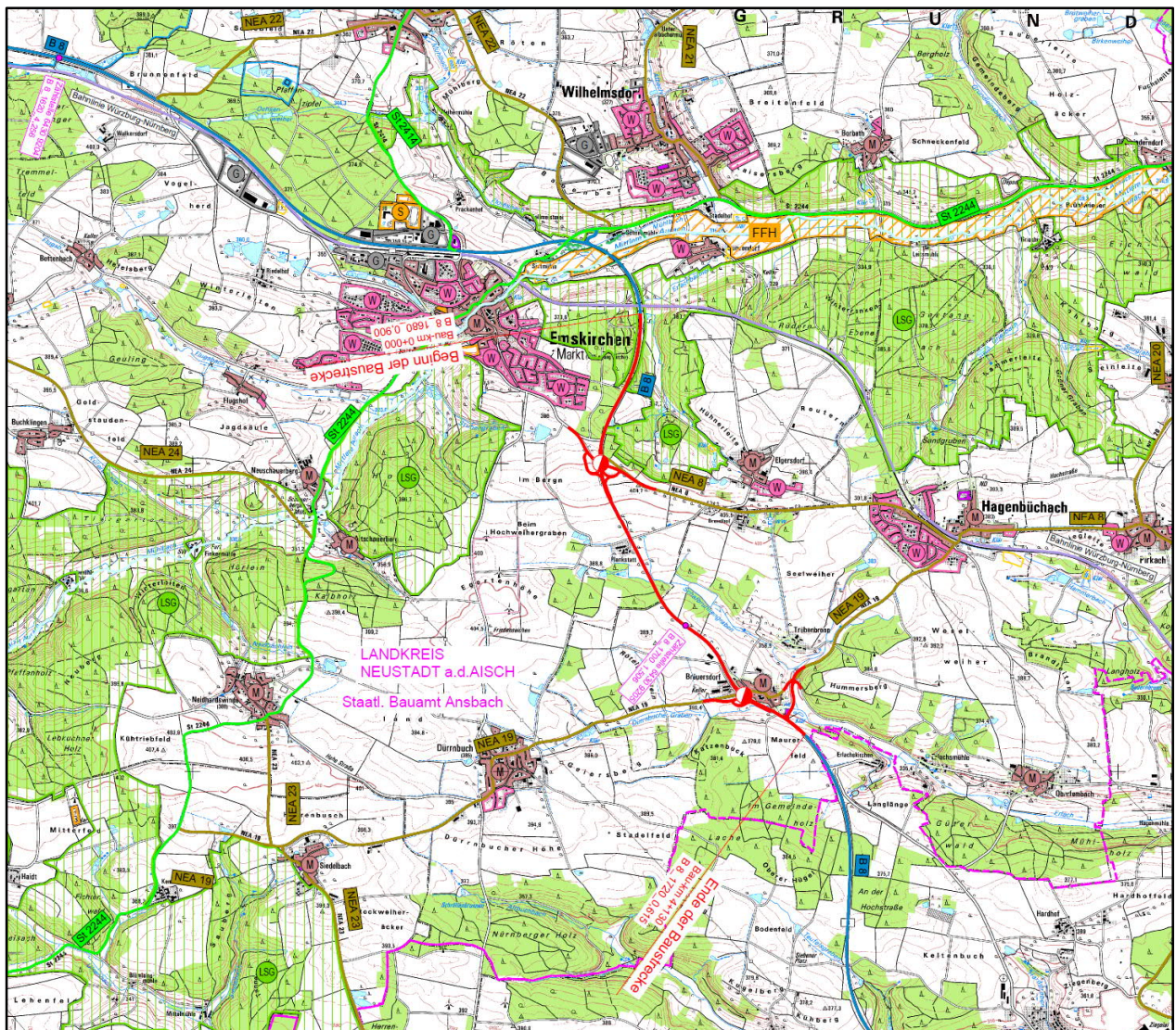
Bild 1: Übersichtslageplan der Maßnahme (unmaßstäblich)
