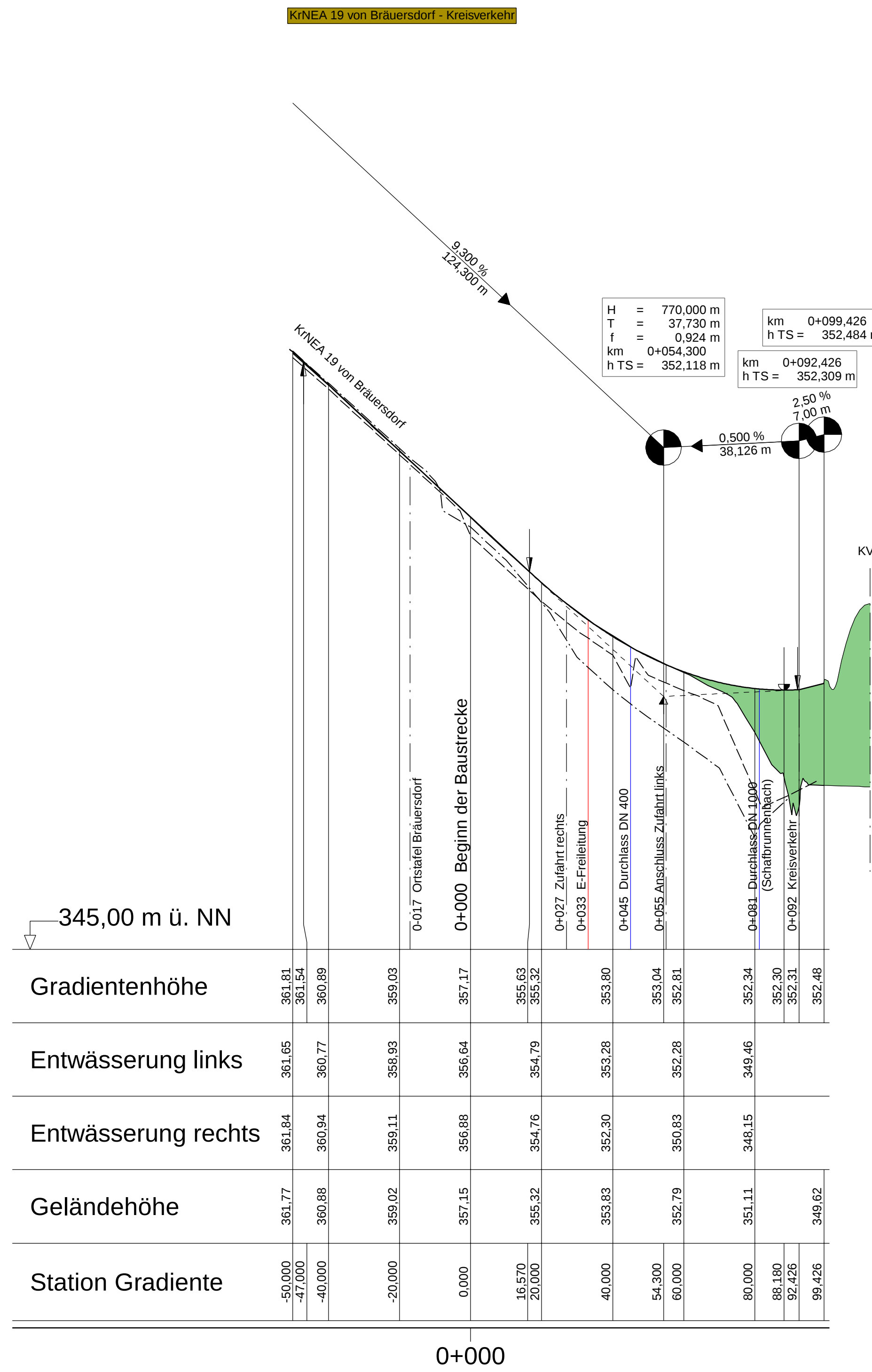
Entwässerungsabschnitt 10
