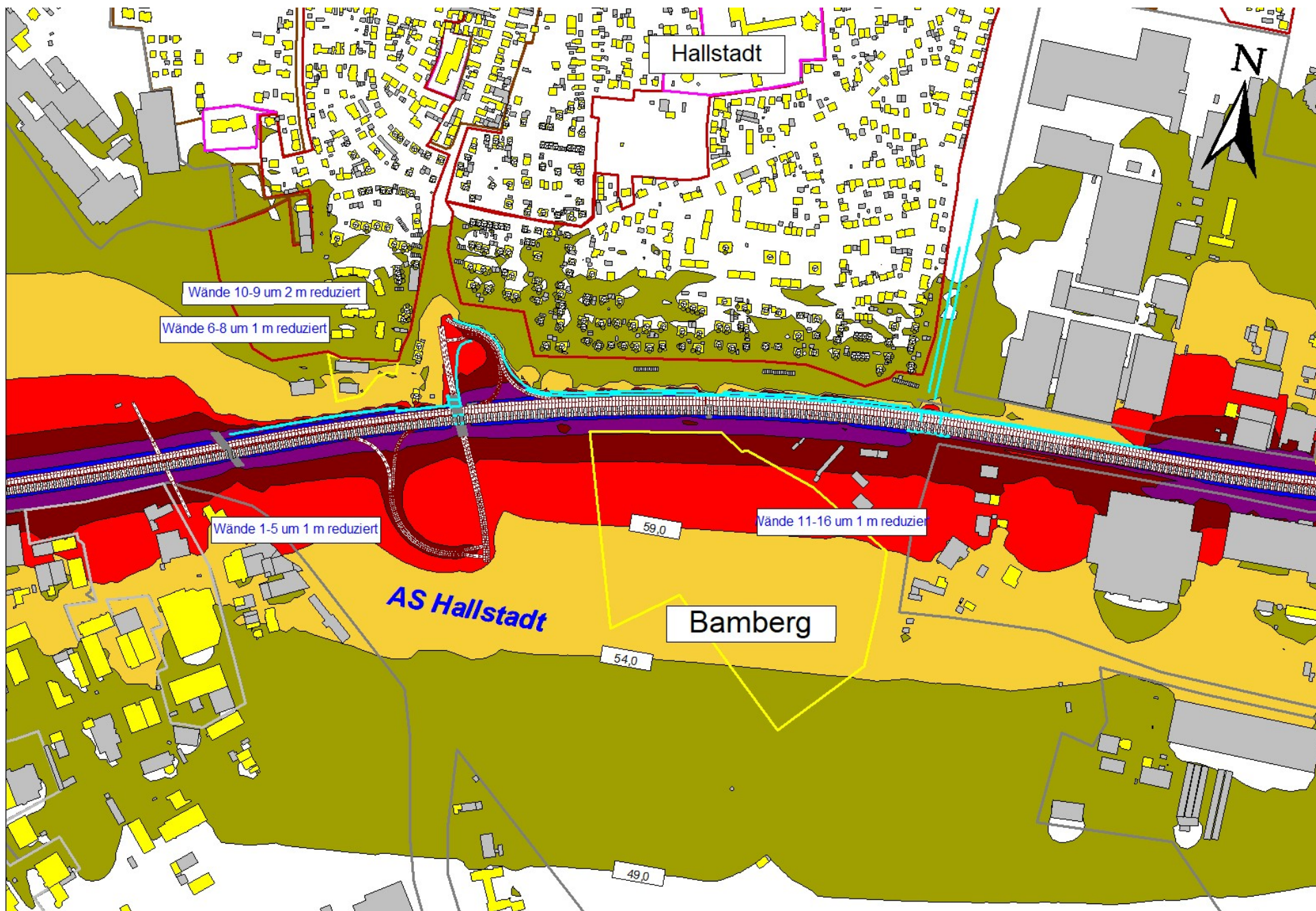
Raster der Isophonen in der Nacht, 6m über Gelände, Variante V 03
