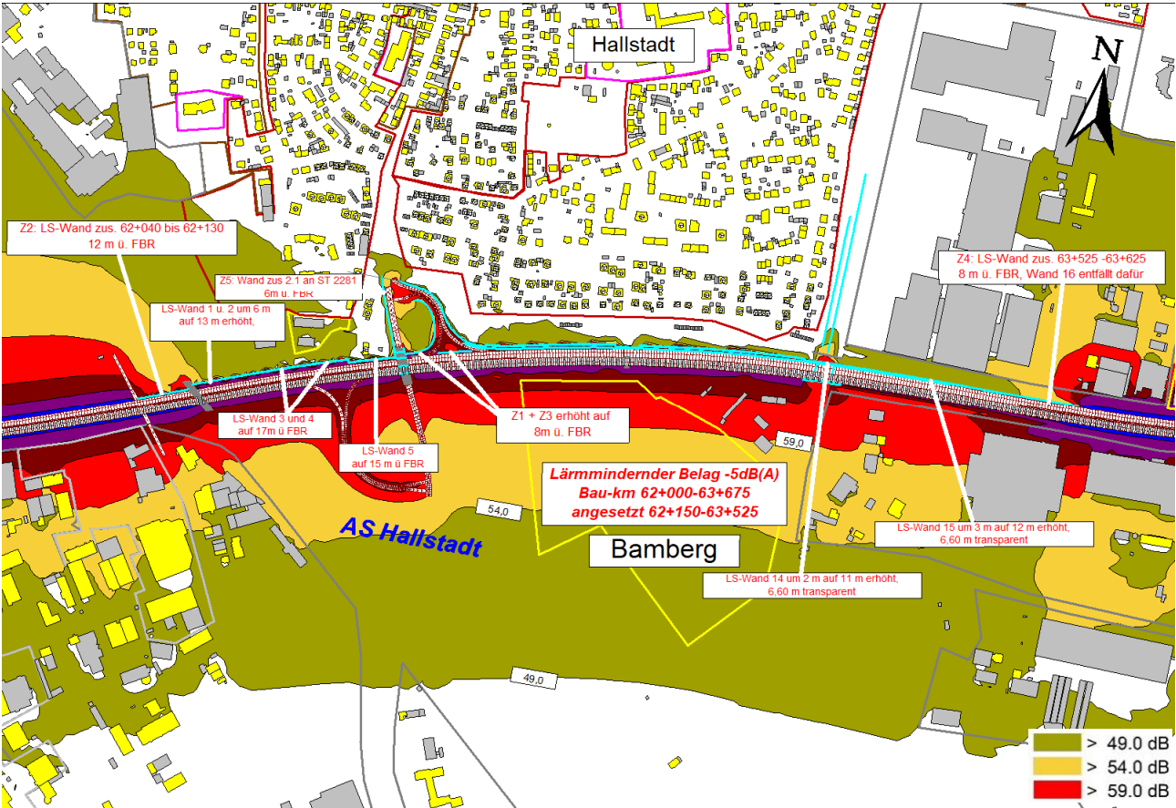
Abb. 9: Variante -06, Raster CadnaA, 6 m ü. Gelände, Isophonen in der Nacht
