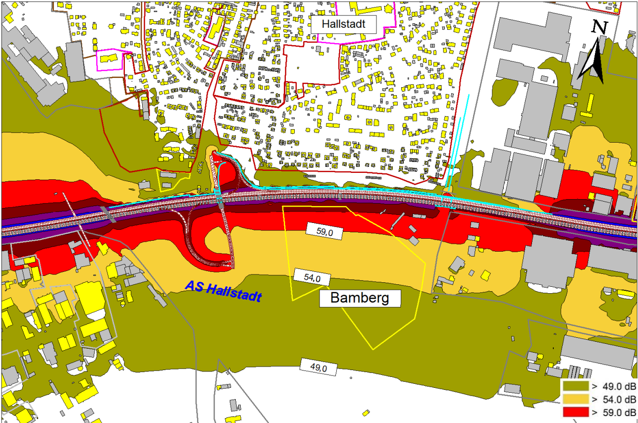
Abb. 7: Variante -04, Raster CadnaA, 6 m ü. Gelände, Isophonen in der Nacht
