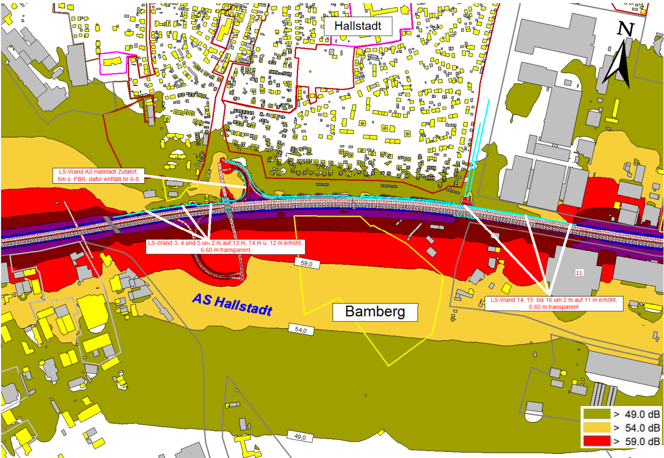
Abb. 5: Variante -02, Raster CadnaA, 6 m ü. Gelände, Raster CadnaA, 6 m ü. Gelände, Isophonen in der Nacht
