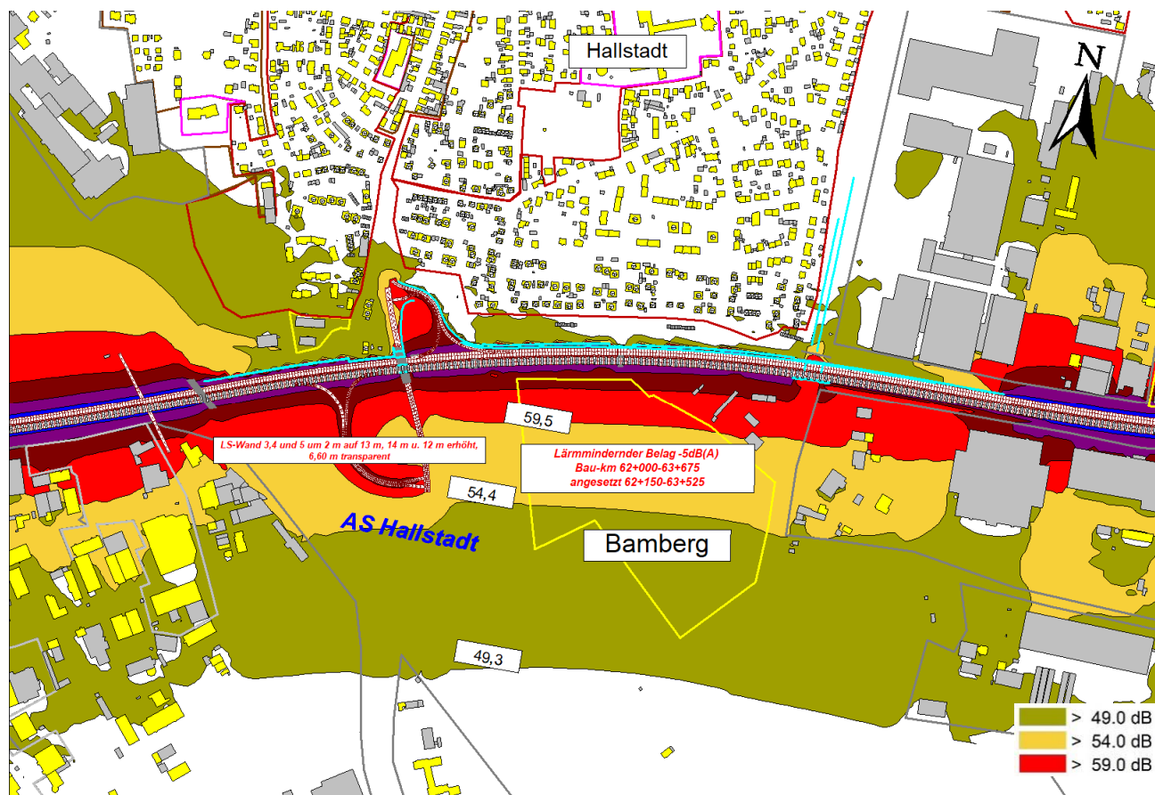
Abb. 8: Variante -05, Raster CadnaA, 6 m ü. Gelände, Isophonen in der Nacht
