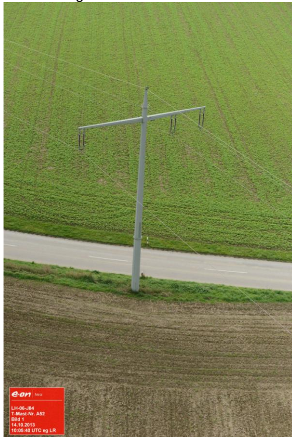
Foto 24: Ltg- Nr. J84 – Mast Nr. A52
