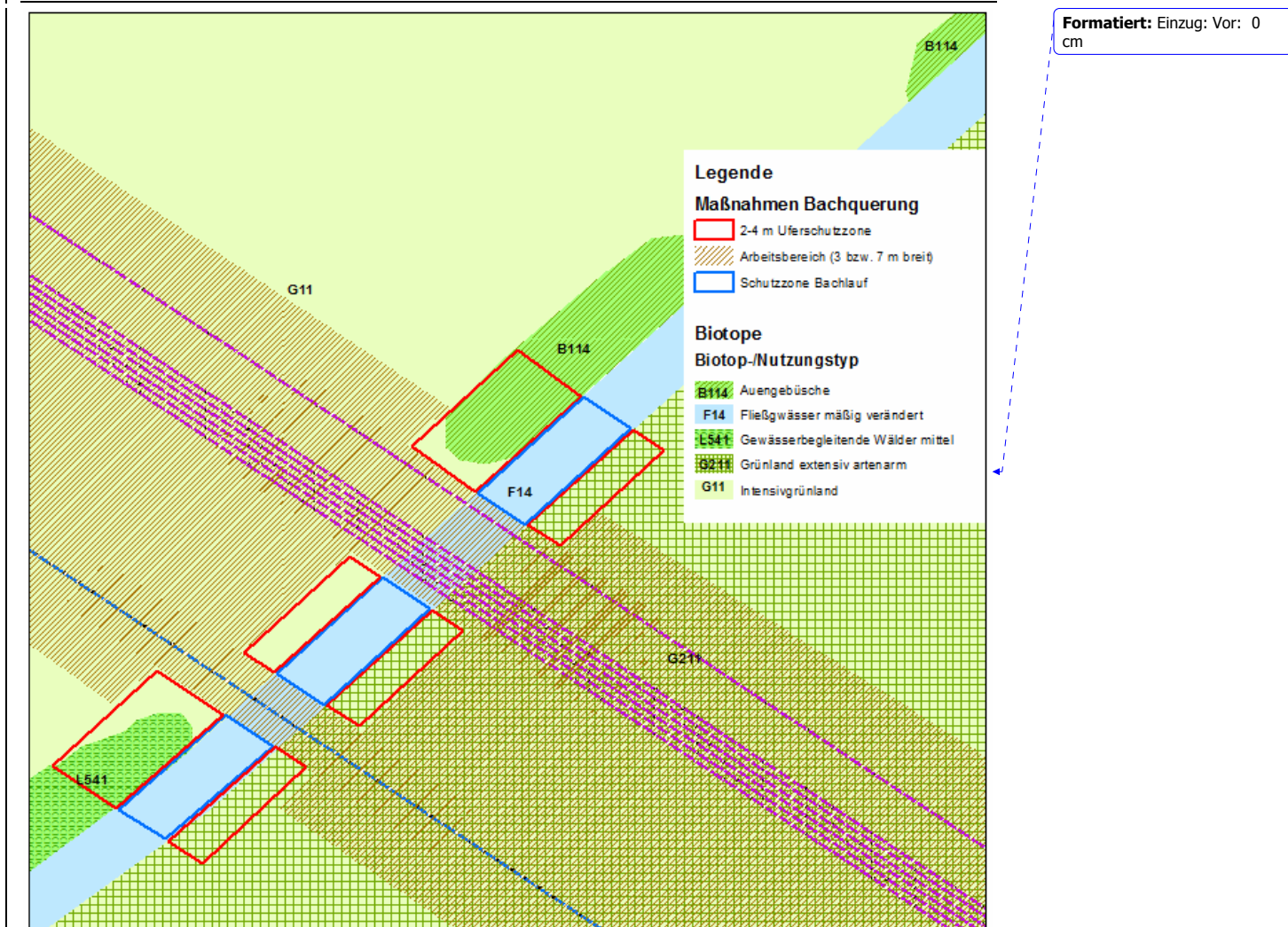
Abb. 2: Schematische Darstellung der Maßnahme V5 (soweit flächig darstellbar) im Bereich des Bubesheimer Bachs (blau = Gasleitung, lila = Stromleitungen).
