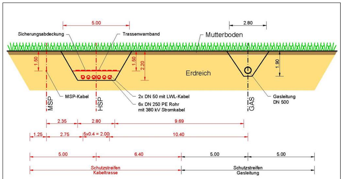
Abbildung 19. Regelgrabenprofil für die Erdkabeltrasse (Quelle: K2 Engineering GmbH)
