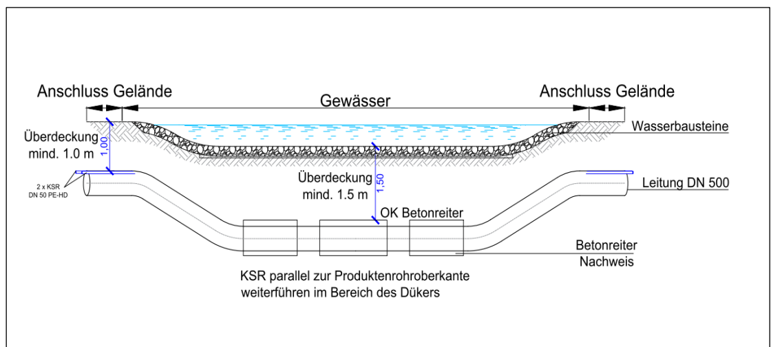
Abbildung 5. Offene Gewässerquerung mittels Düker (Quelle: Ingenieur- und Planungsbüro Lange GbR)
