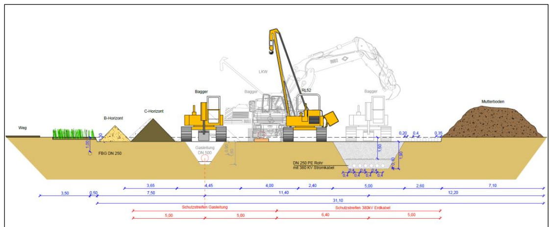
Abbildung 20. Flächenbedarf offene Bauweise bei gemeinsamer Ausführung der AL GKL und des Erdkabels GKL (Quelle: K2 Engineering GmbH)
