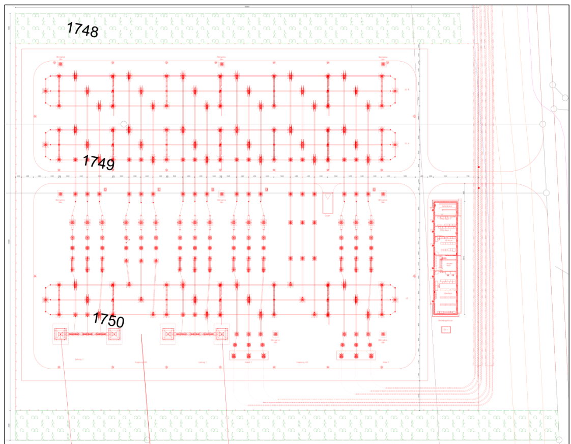
Abbildung 21. Schaltanlage – Draufsicht (Quelle: SPIE SAG GmbH, SAB Oberhausen)
