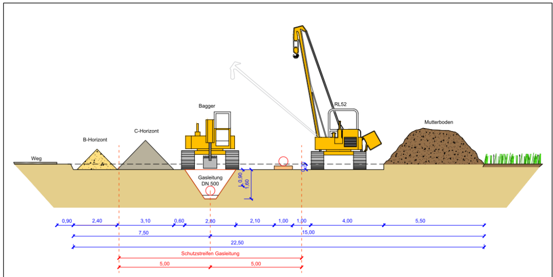
Abbildung 3. Regelarbeitsstreifen im freien Gelände (Quelle: Ingenieur- und Planungsbüro Lange GbR)
