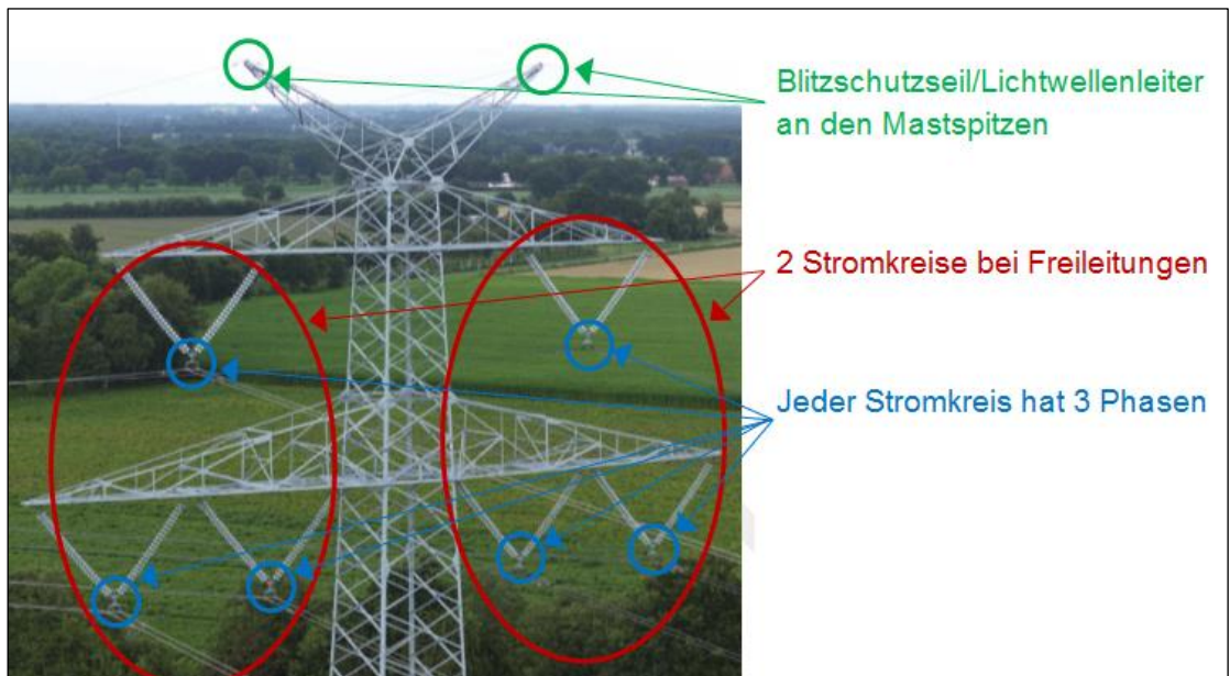
Abbildung 24. Beispiel einer 380-kV-Leitungsbesilung an einem Donaumast mit V-Ketten (Quelle: K2 Engineering GmbH)
