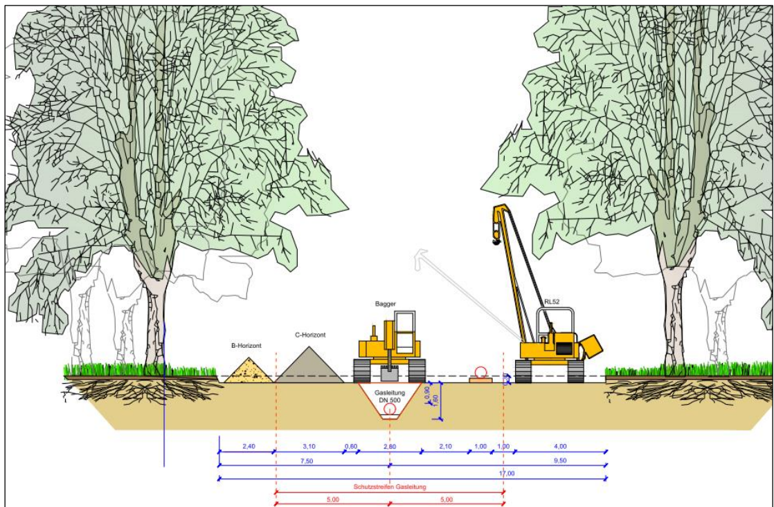
Abbildung 4. Regelarbeitsstreifen im Wald (Quelle: Ingenieur- und Planungsbüro Lange GbR)
