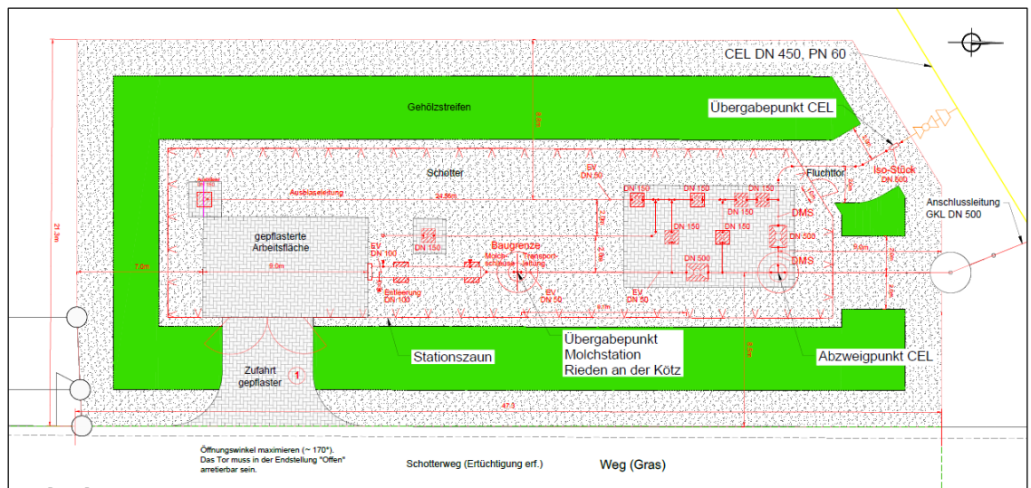
Abbildung 2. Schematische Darstellung der Molchstation Rieden an der Kötz (Quelle: Ingenieur- und Planungsbüro Lange GbR)
