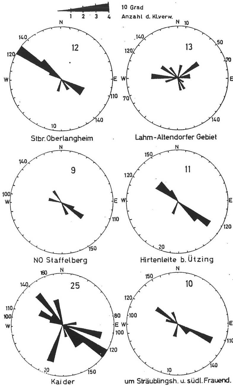
Abb. 14. Kleinverwerfungen.
