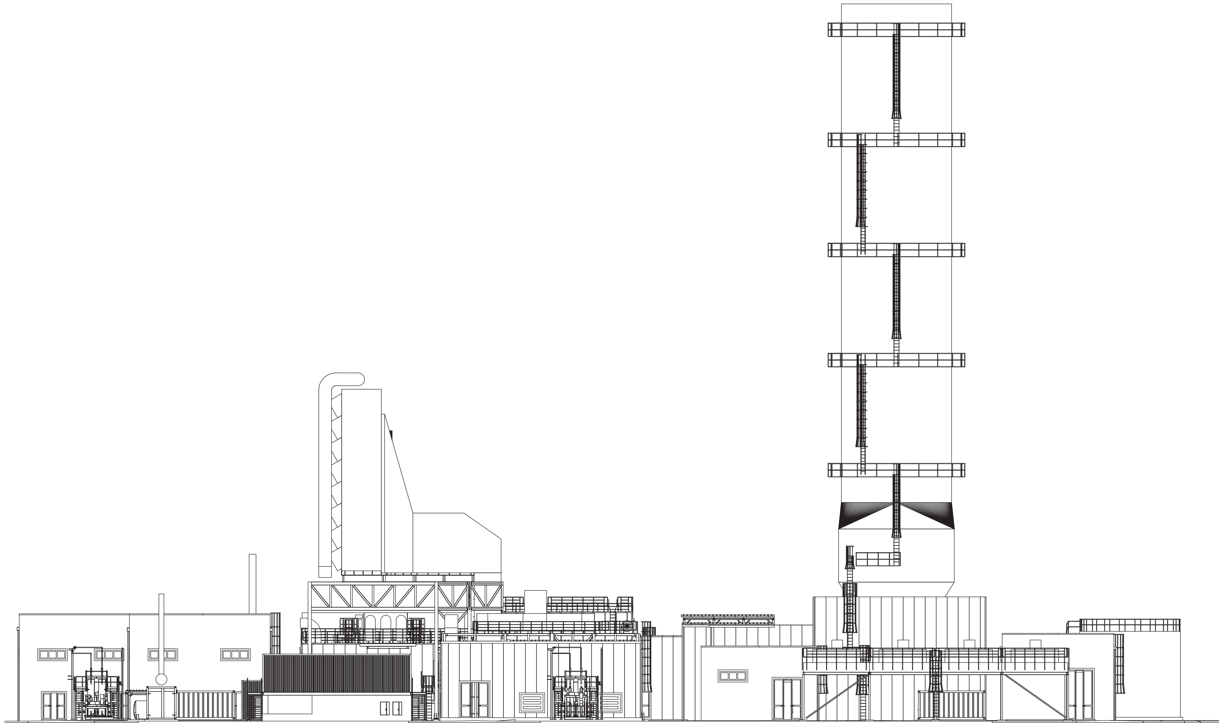
ANSICHT WESTSEITE MAßSTAB 1:200
