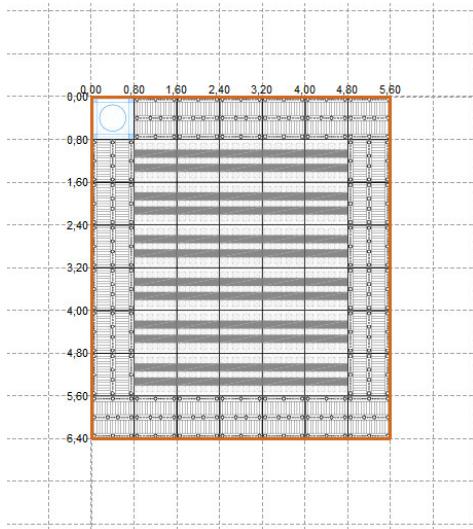
Ebene 1 von Rigole RIG0
