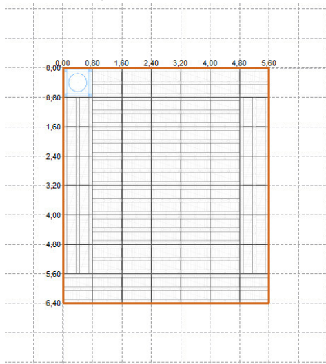
Ebene 3 von Rigole RIG0
