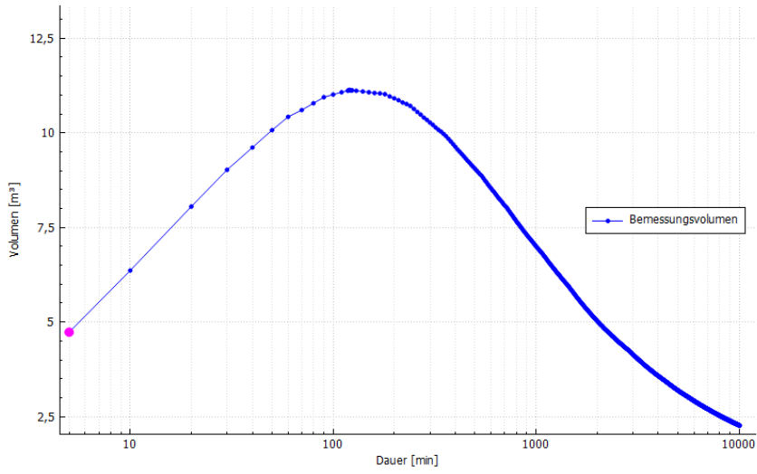
Bemessungskurve von Element WG Mittel
