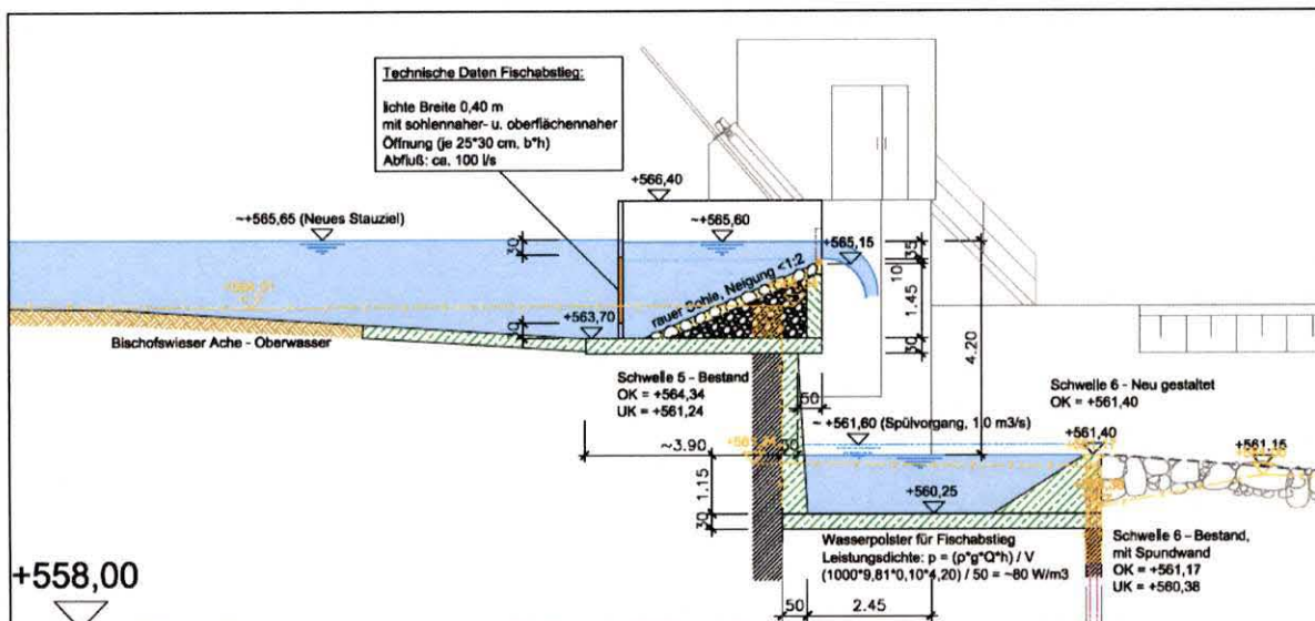
Abbildung 5: Schnitt Fischabstieg - Planung (Auszug aus der Planung von Ederer 2018)
