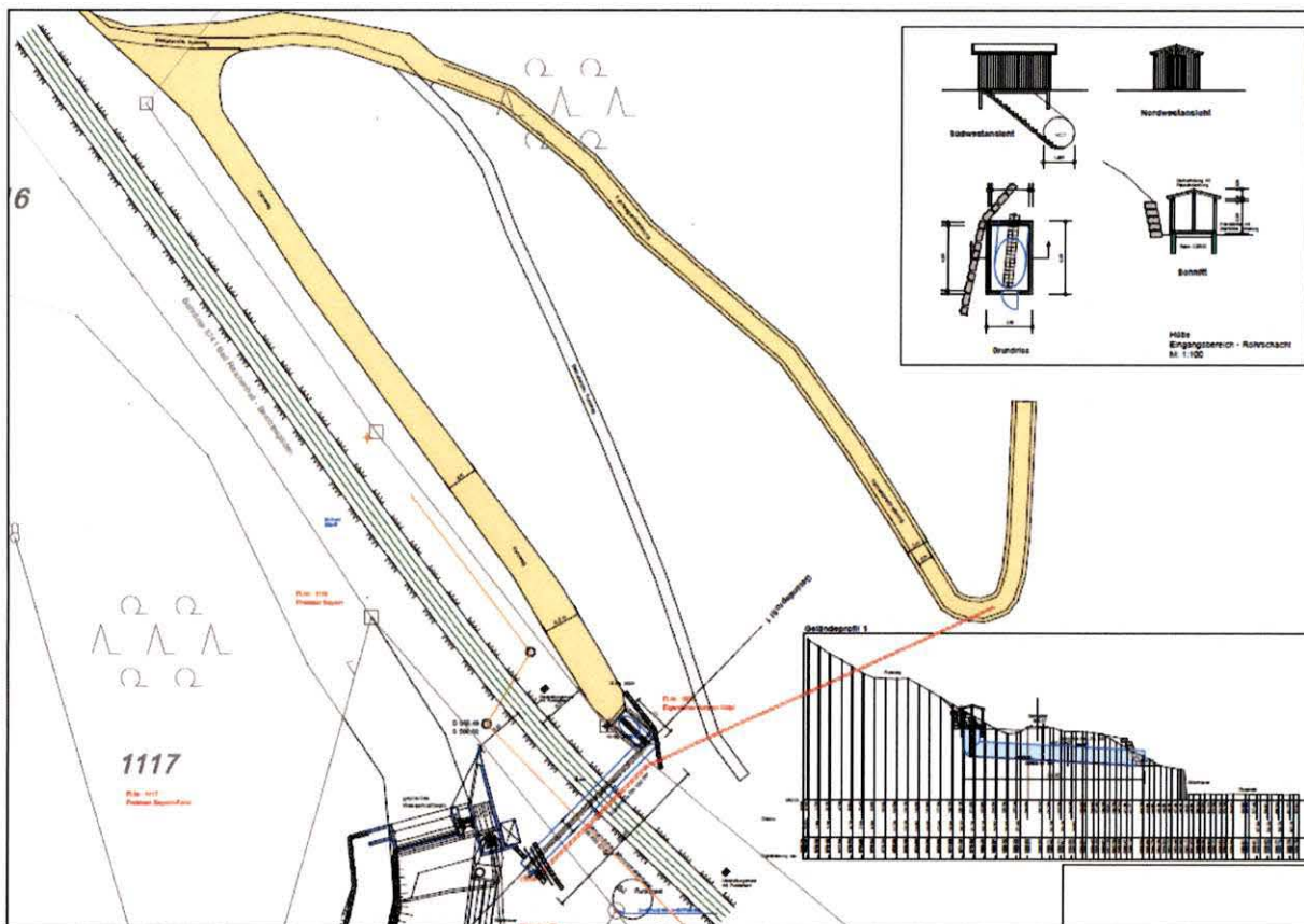
Abbildung 6: Lageplan mit Schnitten Zuwegung, Bahnrohrunterquerung und Holzgebäude oberer Zugang – Planung (IB Liebl 2014)
