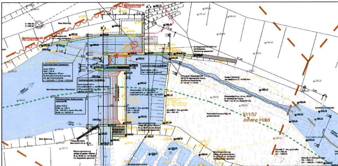
Abbildung 2: Lageplan WKA – Planung (Auszug aus der Planung von Ederer 2018)
