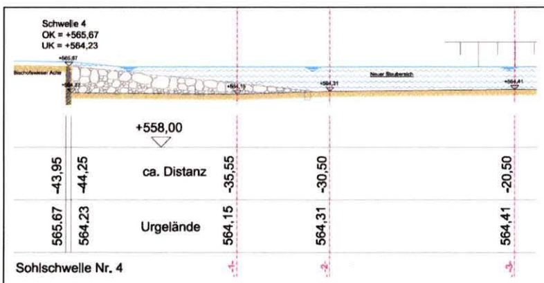
Abbildung 15: Längsschnitt Sohlanrampung (Auszug aus der Planung von Ederer 2018)
