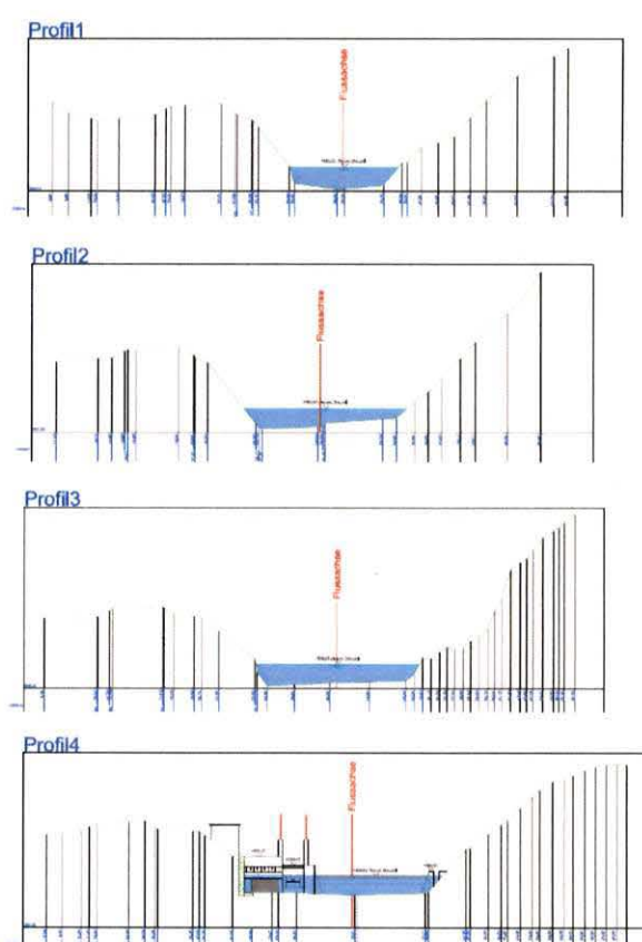
Abbildung 20: Profile im Oberwasser - Planung
