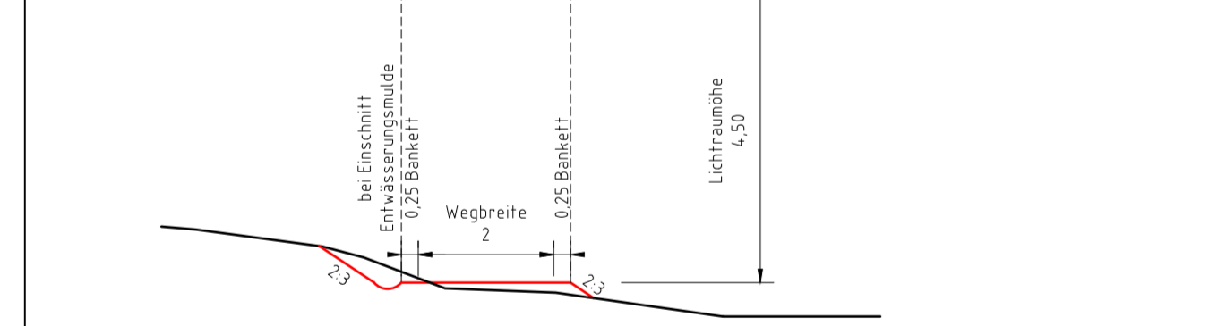
Schema Weg M 1:100
