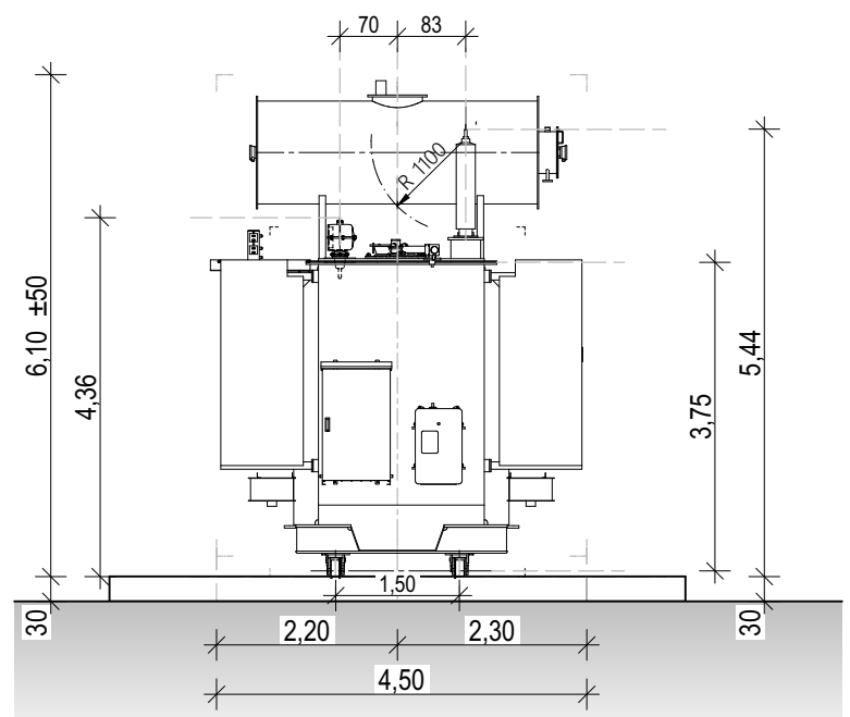
Ansicht Süd
