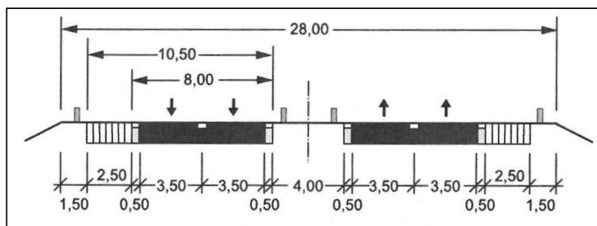
Abb. 14: Regelquerschnitt RQ 28
