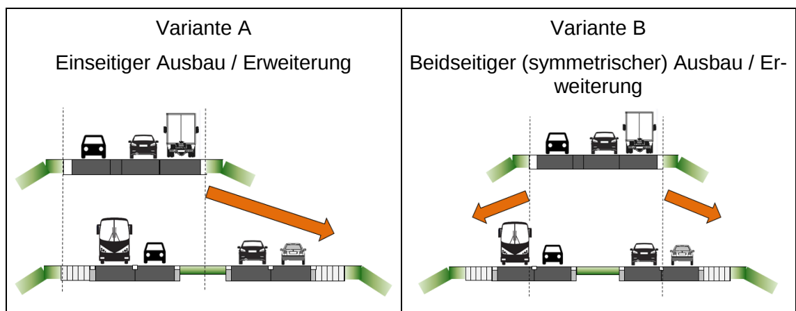
Abb. 4: Ausbauvarianten A und B im Querschnitt
