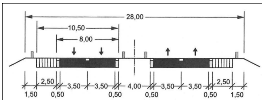
Abb. 2: Regelquerschnitt RQ28
