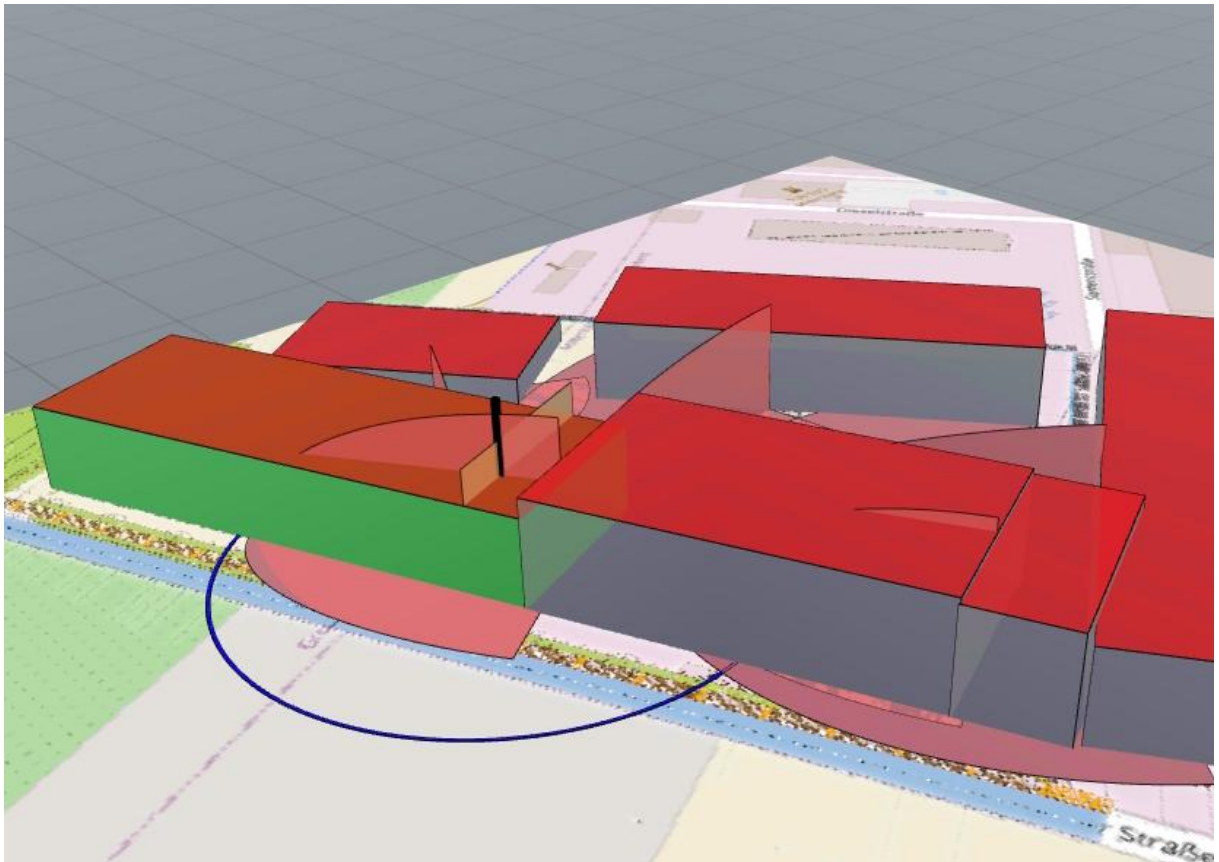
Abbildung 5: Störzonen und Einwirkbereich PM8_02 (Staubabsaugung)
