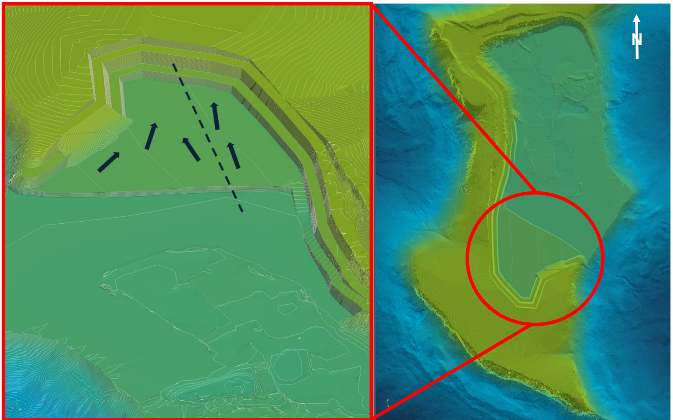
Abb. 27: Darstellung der geplanten Wasserführung in der Erweiterungsfläche. Zu sehen ist a) die Neigung der Tiefsohle in Richtung Süden und b) die Modellierung entlang der vor dem Abbau existierenden oberflächlichen Wasserscheide (gestrichelte Linie). Dadurch soll das anfallendes Oberflächenwasser wirksam in dem Erweiterungsbereich zurückgehalten werden (angedeutet durch Pfeile). Auf dieser Fläche wird zudem die Rekultivierungsschicht hergestellt (Bild: Fa. Holcim).
