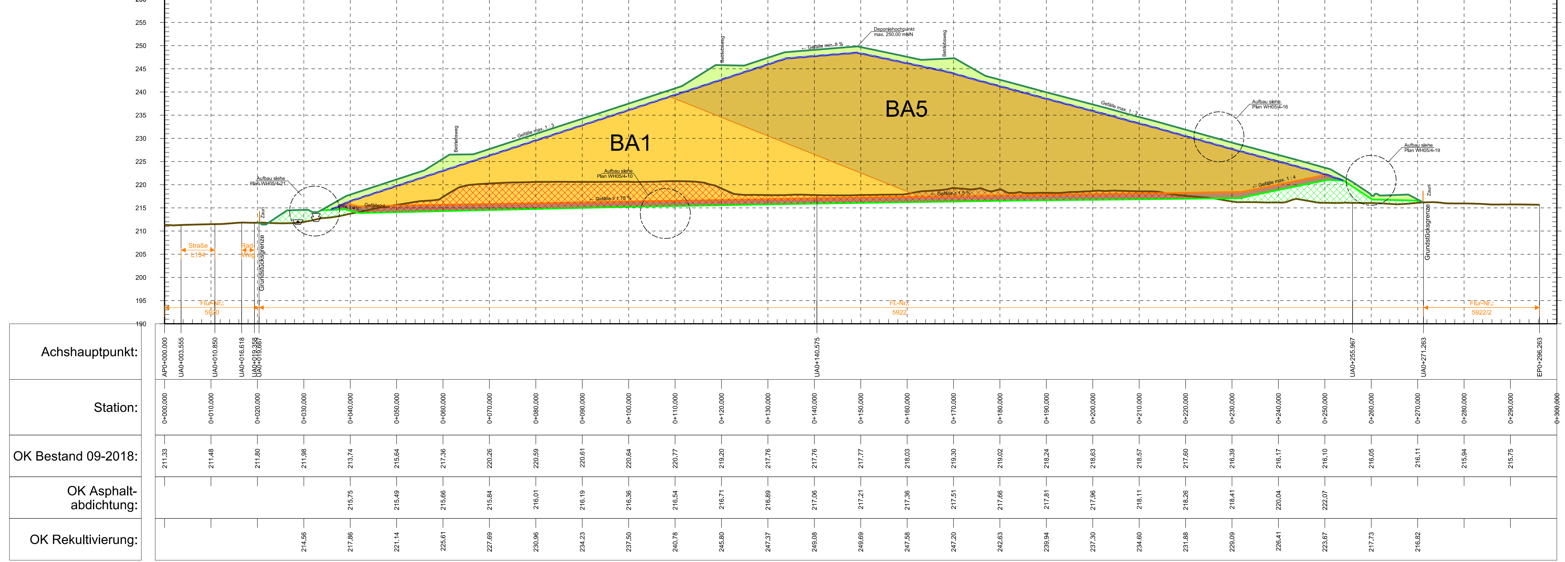
Längsschnitt 3 - 3
