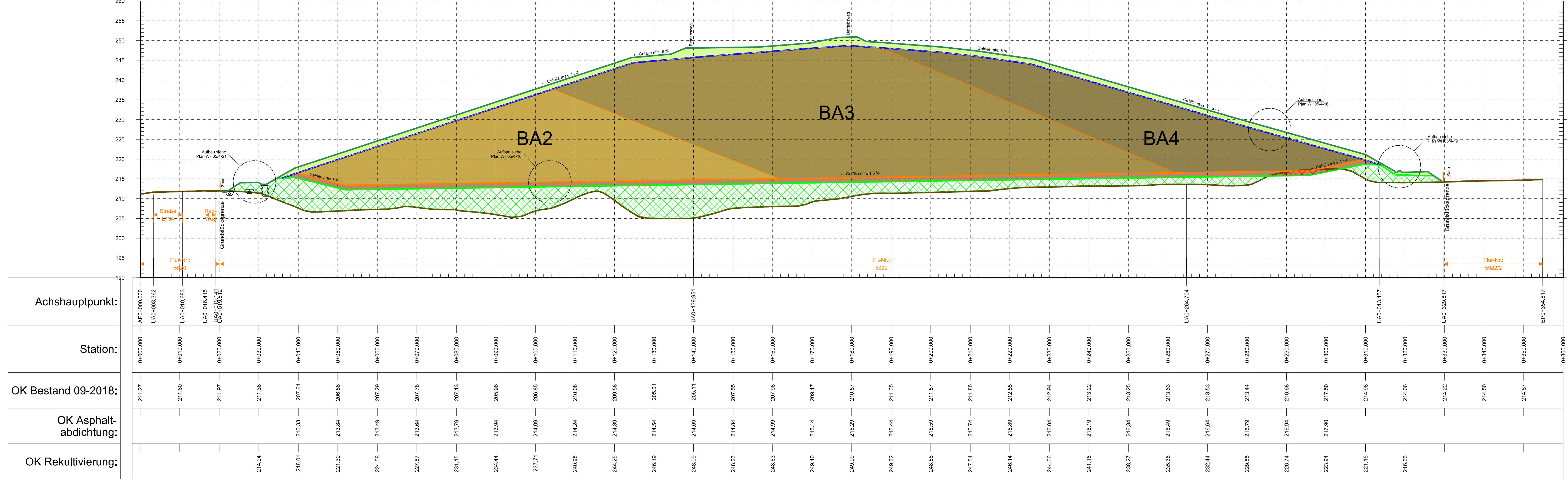
Längsschnitt 2 - 2
