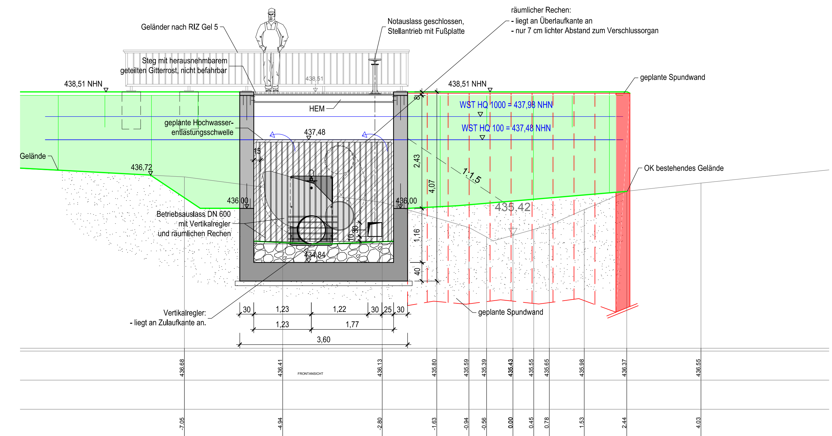
Schnitt B - B
