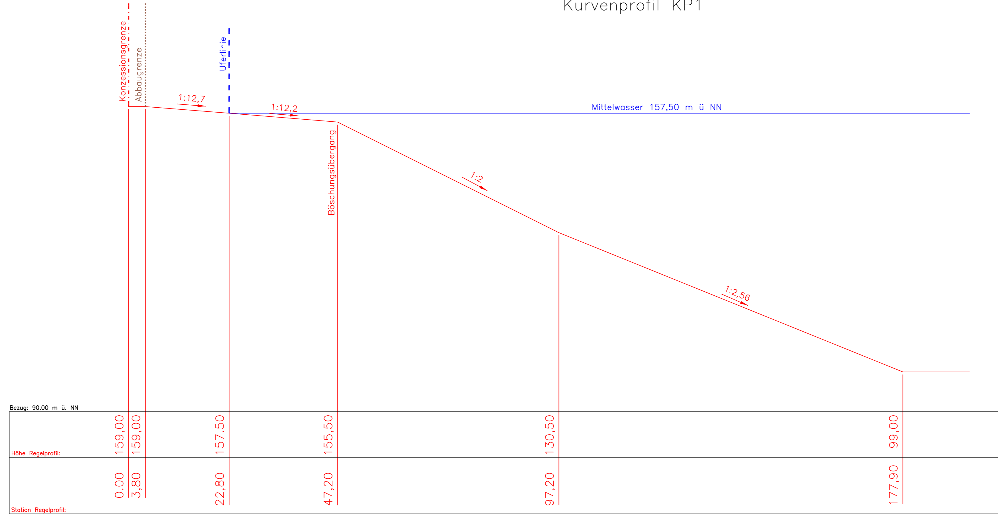
Kurvenprofil KP1
