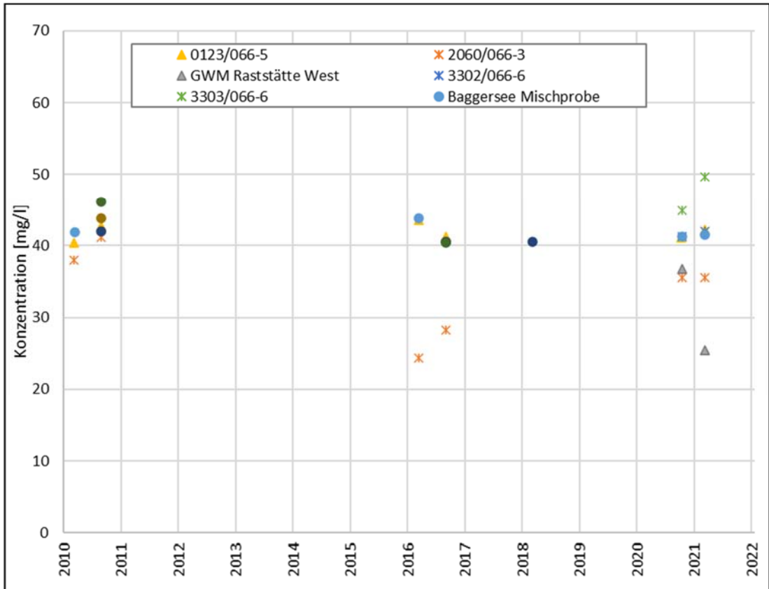
Abbildung 1: Ergebnisse Chloridanalysen
