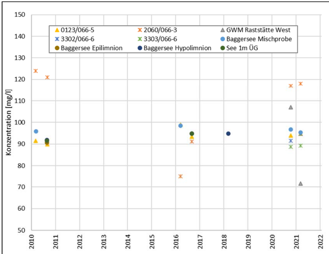
Abbildung 3: Ergebnisse Sulfatanalysen
