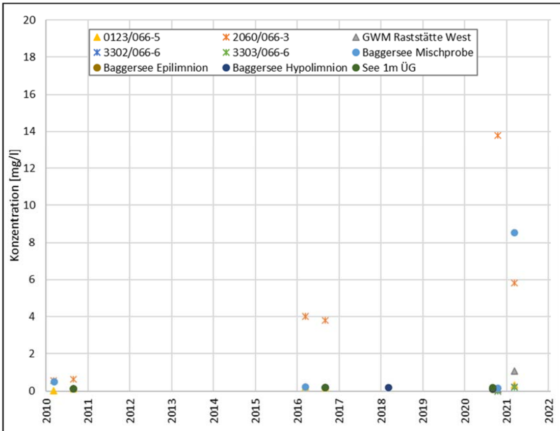
Abbildung 2: Ergebnisse Nitratanalysen
