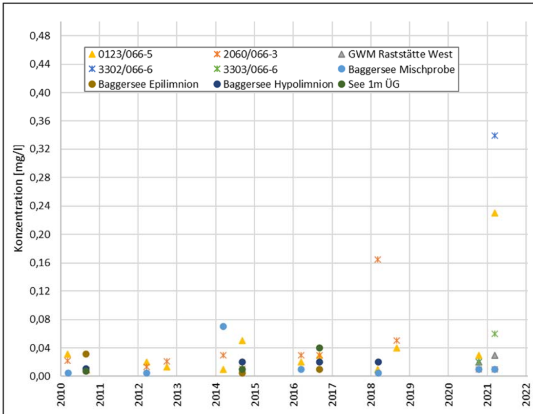
Abbildung 4: Ergebnisse Phosphoranalysen
