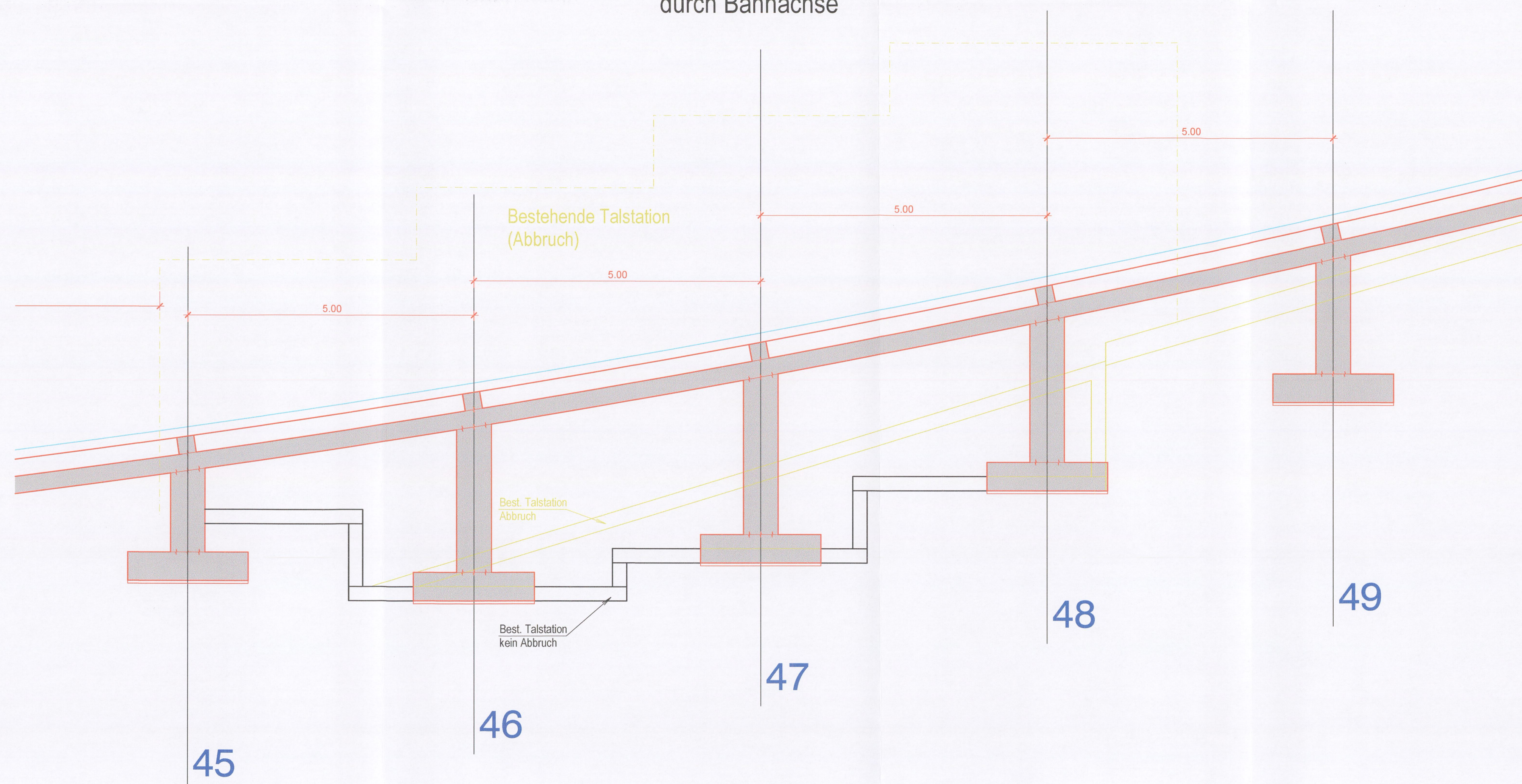
Längsschnitt 1:50 durch Bahnachse
