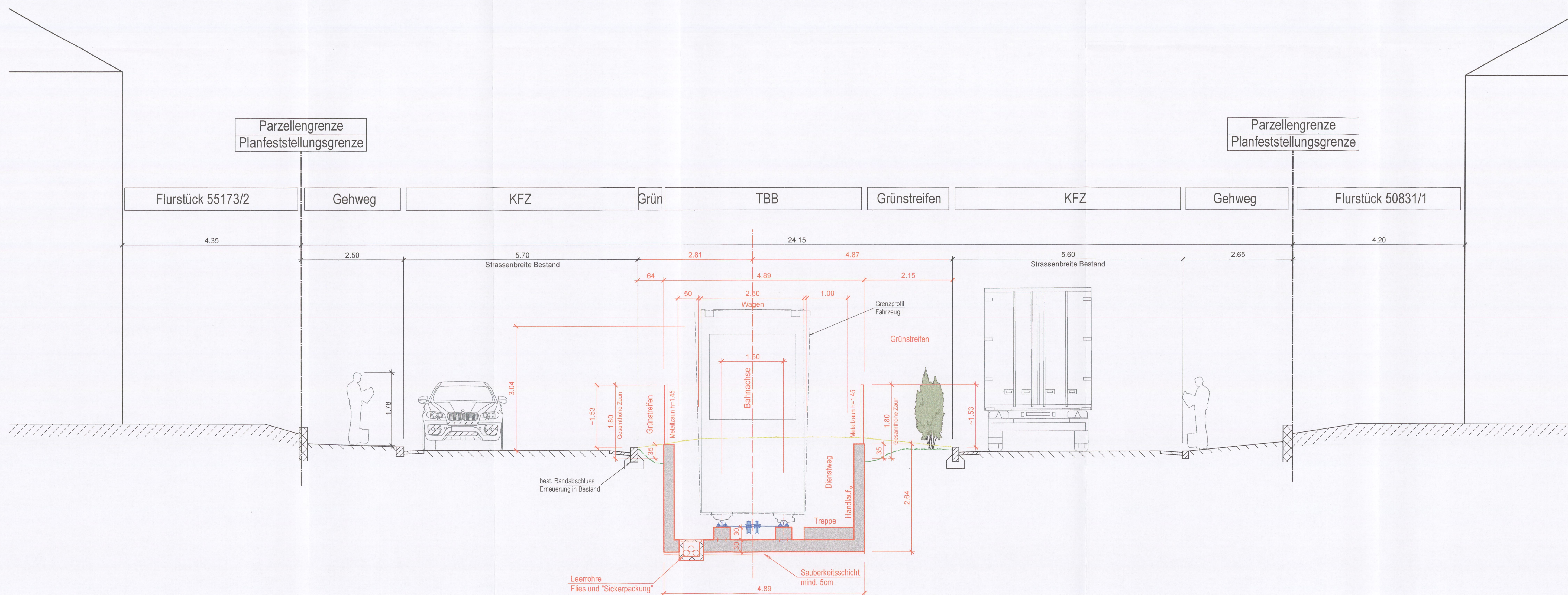
Querprofil 11, 1:50 Km 50.00, Blickrichtung Berg
